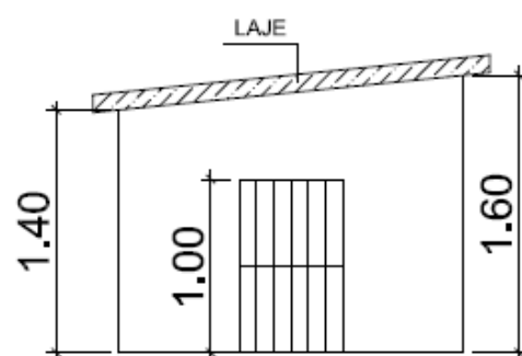
Fachada
