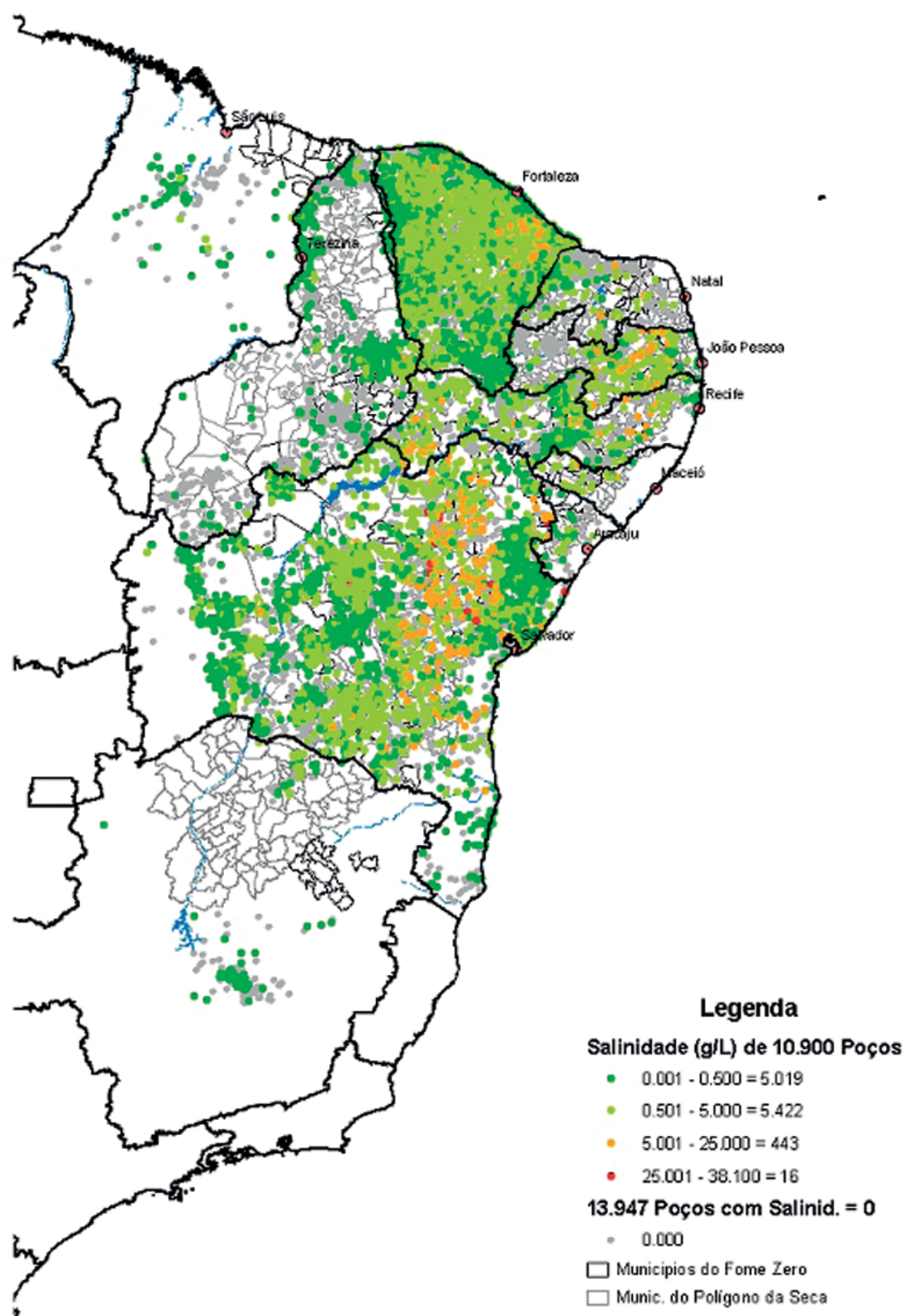
Figura 16: Hierarquização de áreas e poços para implantação de sistemas alternativos de extração de sais Fonte: Embrapa, Meio Ambiente.
