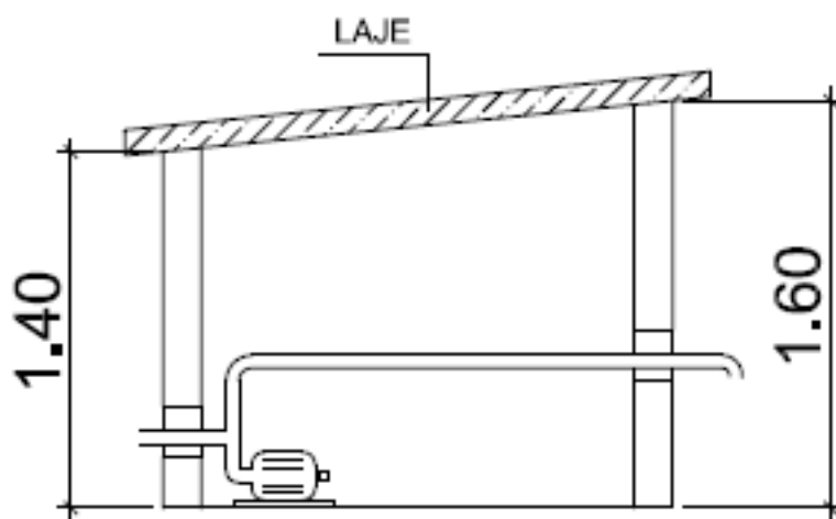
Corte AA'
