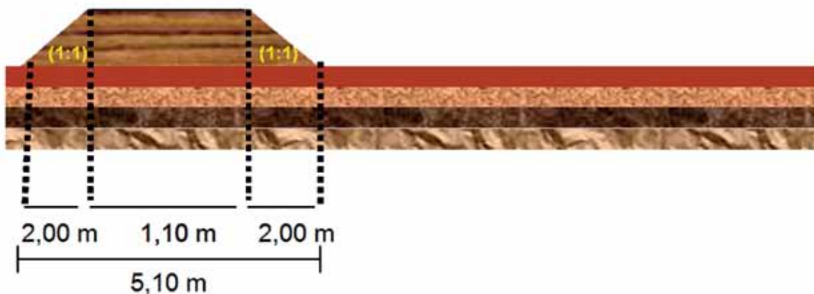
Figura 35 Corte Transversal do tanque de armazenamento de rejeito
