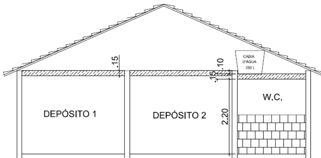
Corte AA'
