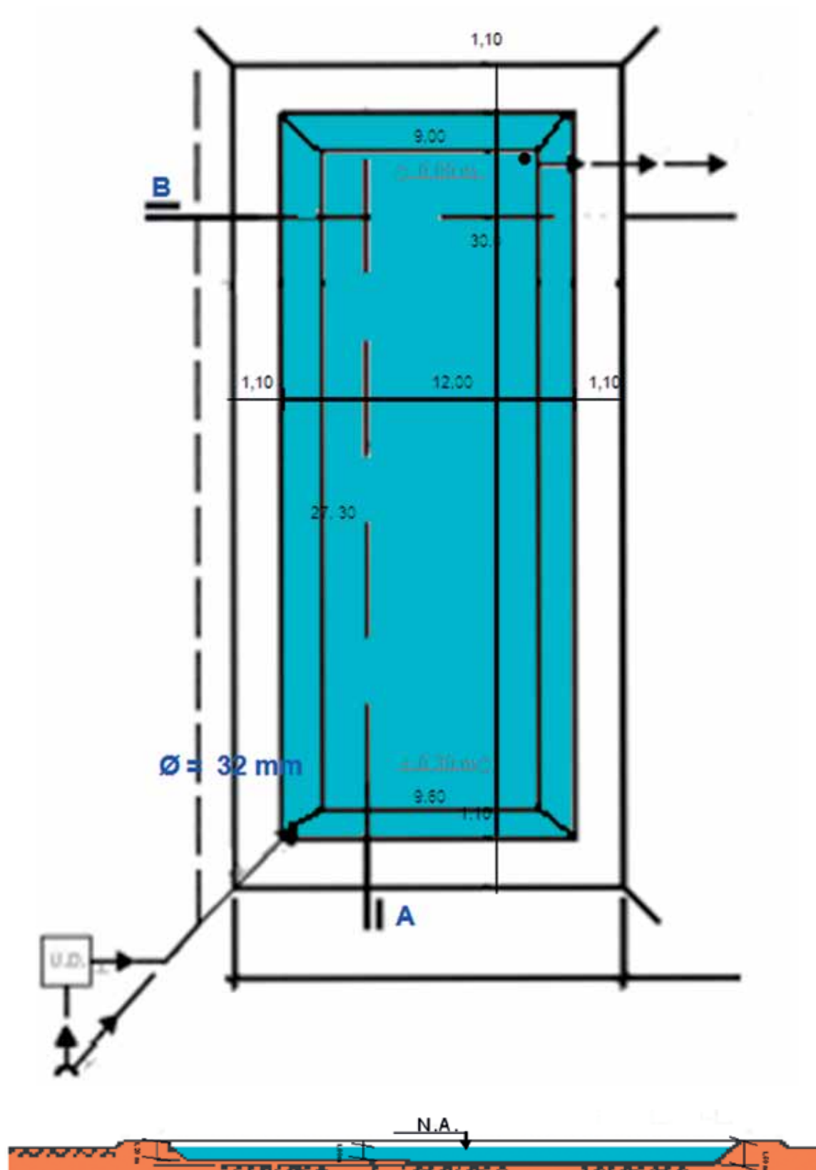
Corte AA'
