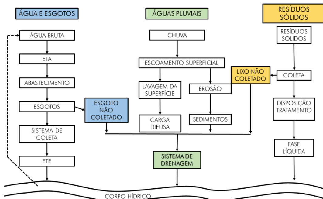
Figura 3.1 - Representação gráfica do fluxo dos esgotos e dos resíduos sólidos não coletados para o sistema de drenagem
