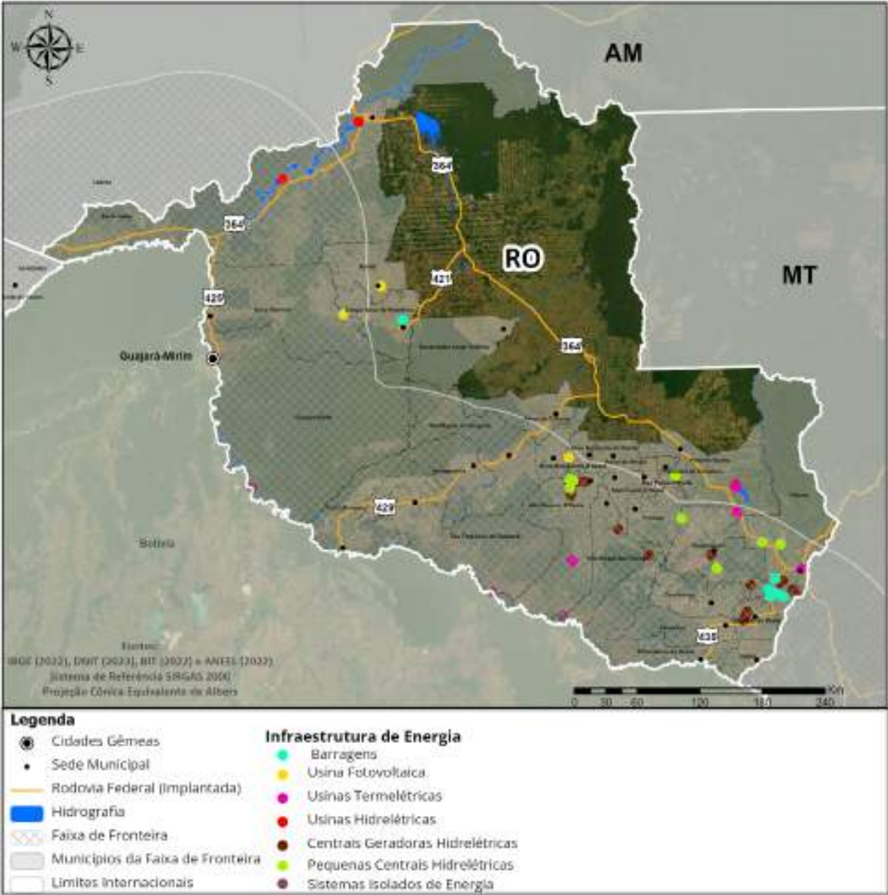
Mapa 6 - Geração de energia elétrica (Infraestrutura de energia e Sistemas Isolados) do Estado de Rondônia
