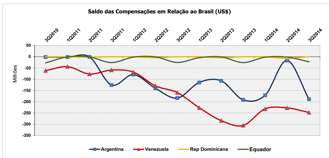
Figura 4 | Saldo das compensações em relação ao Brasil dos 4 países com maiores exposições no FGE em dez/14.
