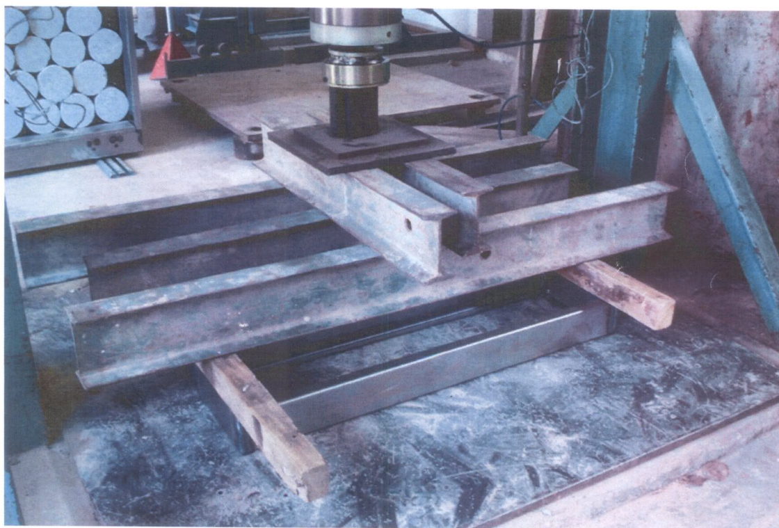
FOTO N.º 02 – SISTEMA DE ENSAIO
