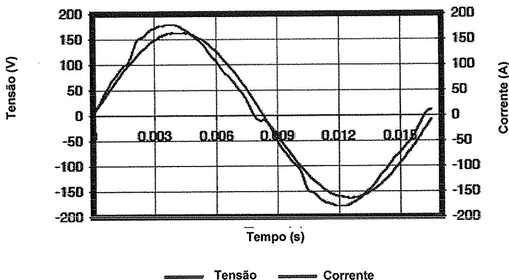
Formato de onda de corrente e tensão de entrada
