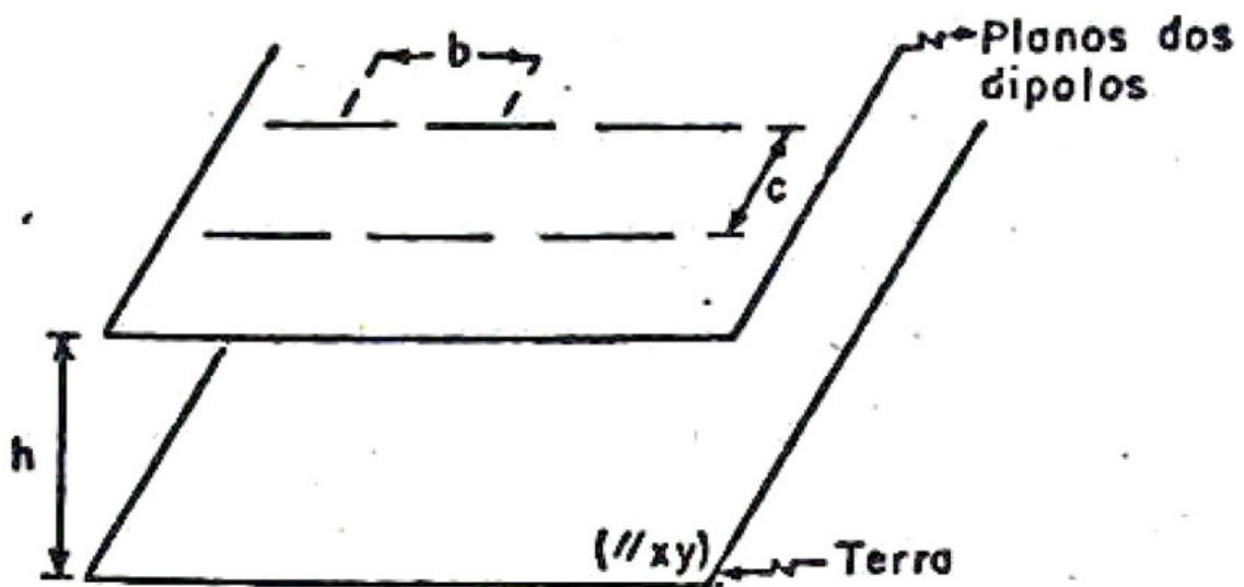
Fig. VII.1 Disposição dos dipolos em uma antena TRO (no caso TRO 3/2\lambda ).
