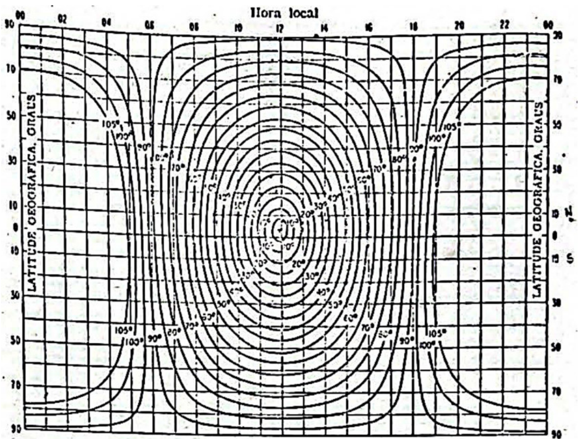
Fig. VI.3 Ângulo zenital do sol, x (junho).
