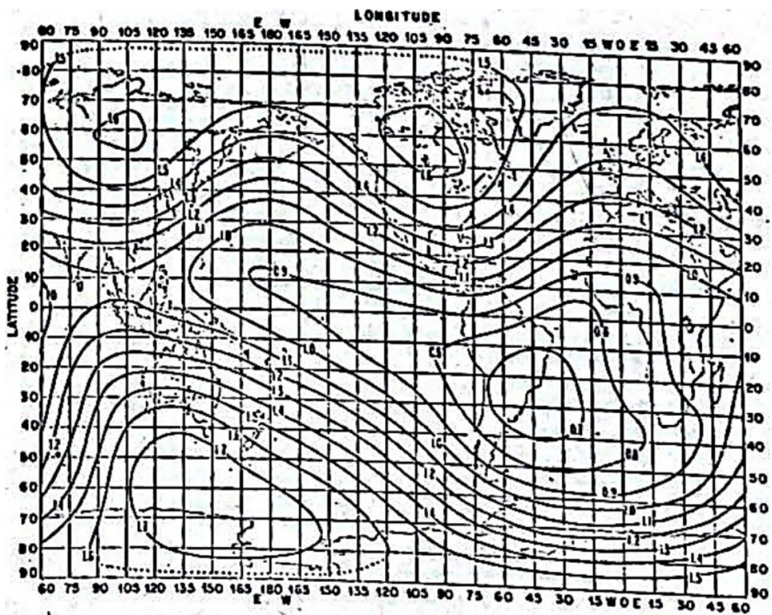
Fig. VI.6 Frequência Giromagnética, f_H , em MHz a uma altura de 100km.
