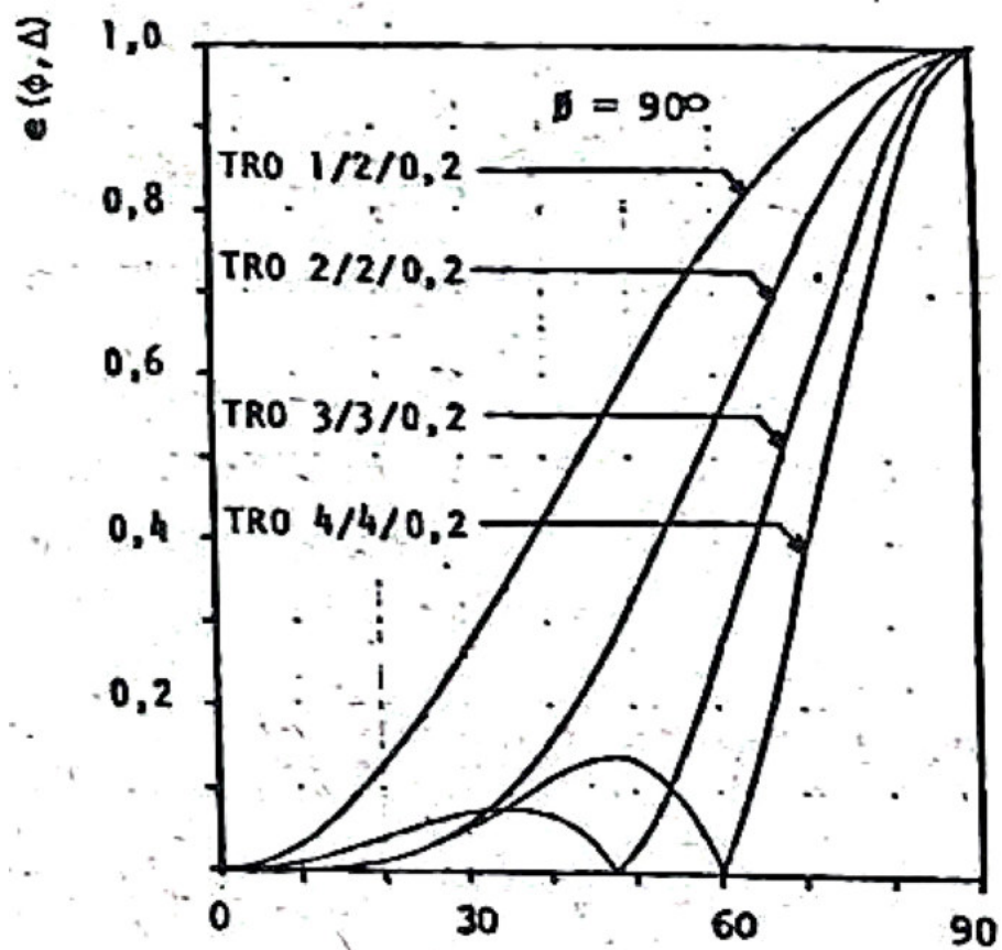
Fig. VII.4 Diagrama Vertical. Antenas tipo TRO.
