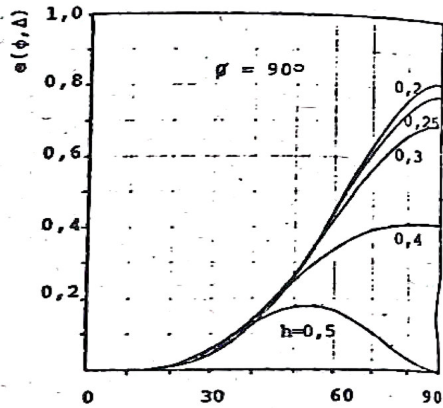
Fig. VII.15 Diagrama Vertical. Antena HR 2/1/\frac{h}{\lambda} . Refletor Ativo.
