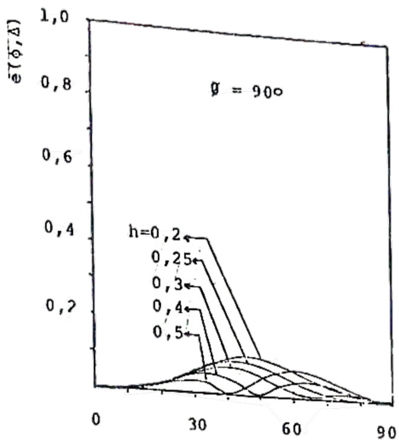
Fig. VII.21 Diagrama Vertical. Antena HR 2/2/\frac{h}{\lambda} . Refletor Ativo.
