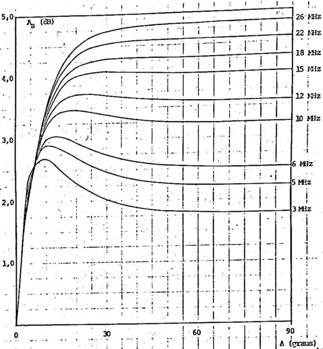
Fig. VI.7 Perda por reflexão no solo, A_s
