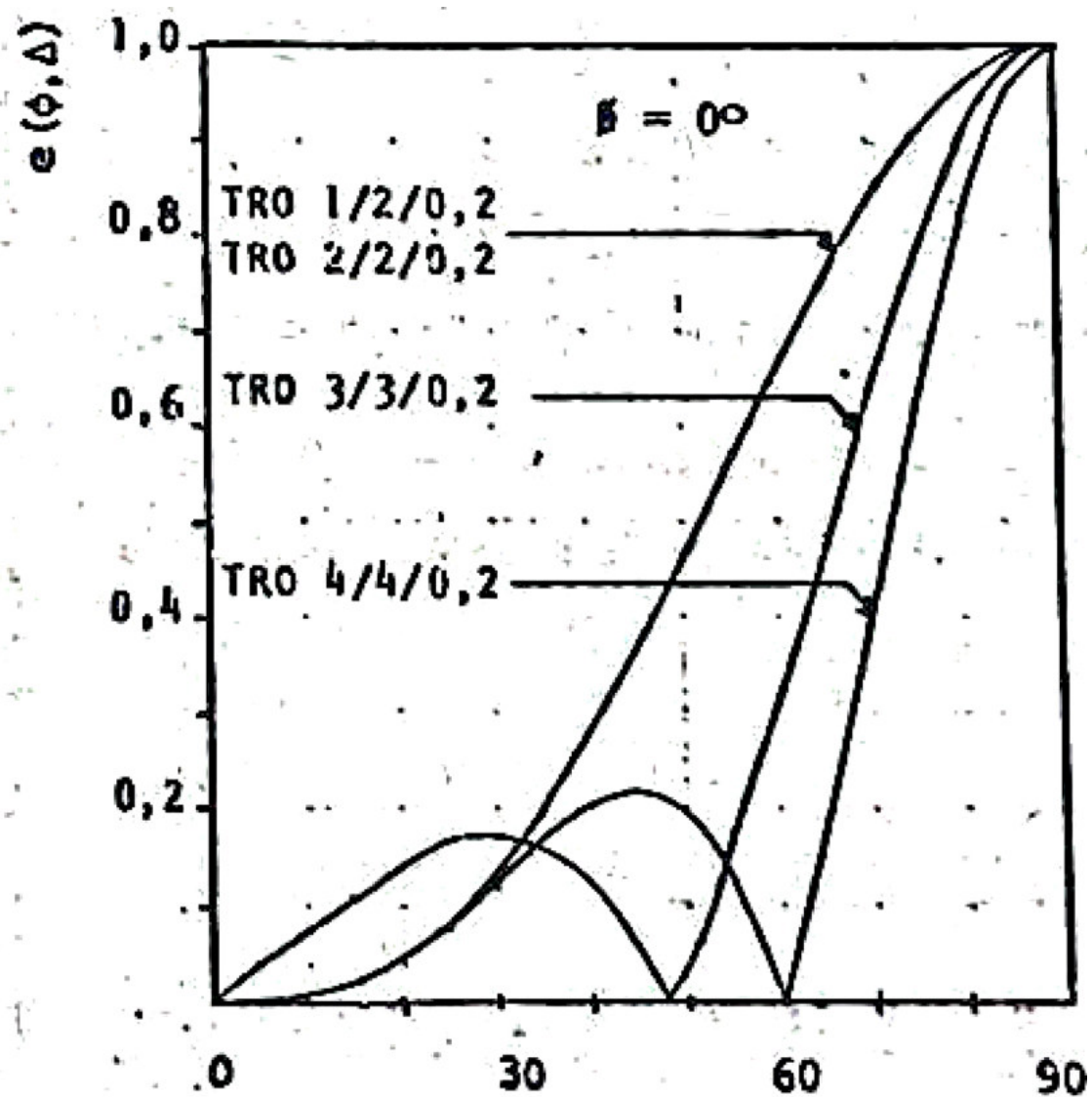
Fig. VII.3 Diagrama Vertical. Antenas tipo TRO.
