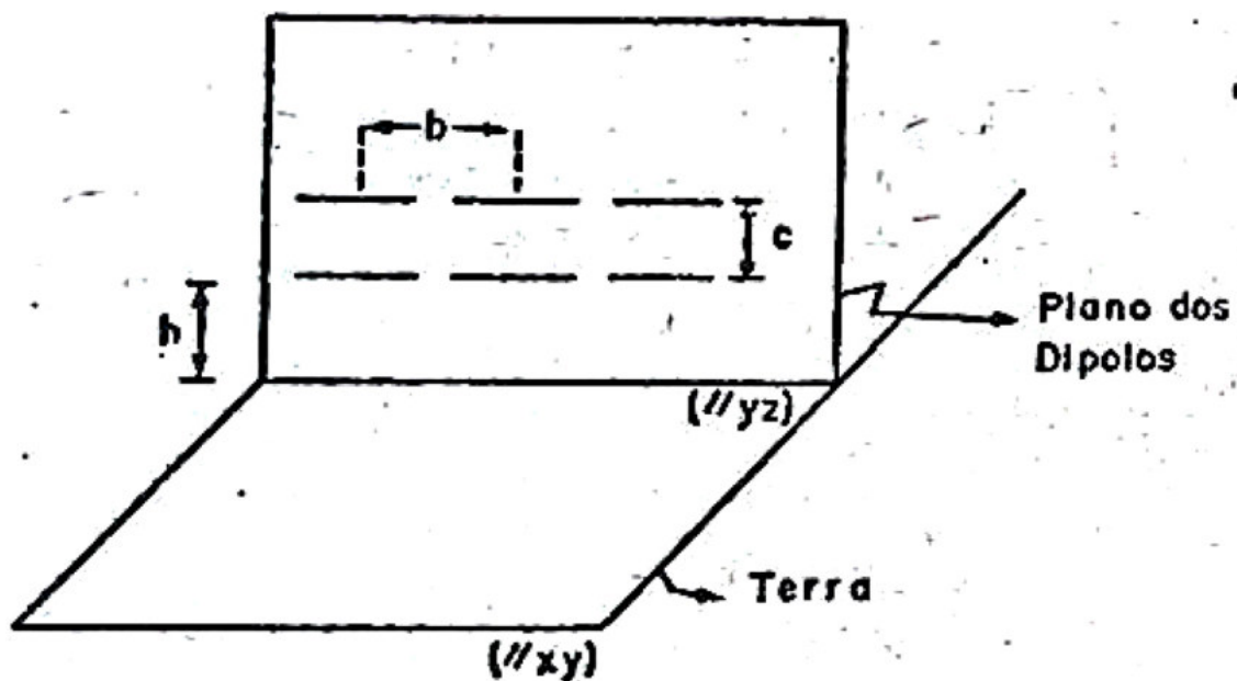
Fig. VII.7 Disposição dos dipolos em uma antena H (no caso, uma H 3/2 \frac{h}{\lambda} ).
