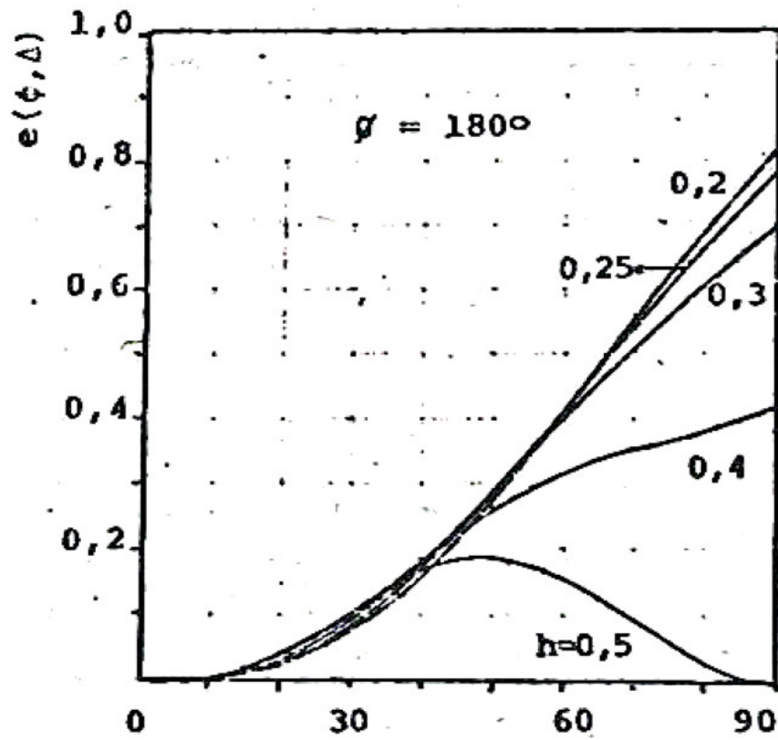
Fig. VII.16 Diagrama Vertical. Antena HR 2/1/\frac{h}{\lambda} . Refletor Ativo.
