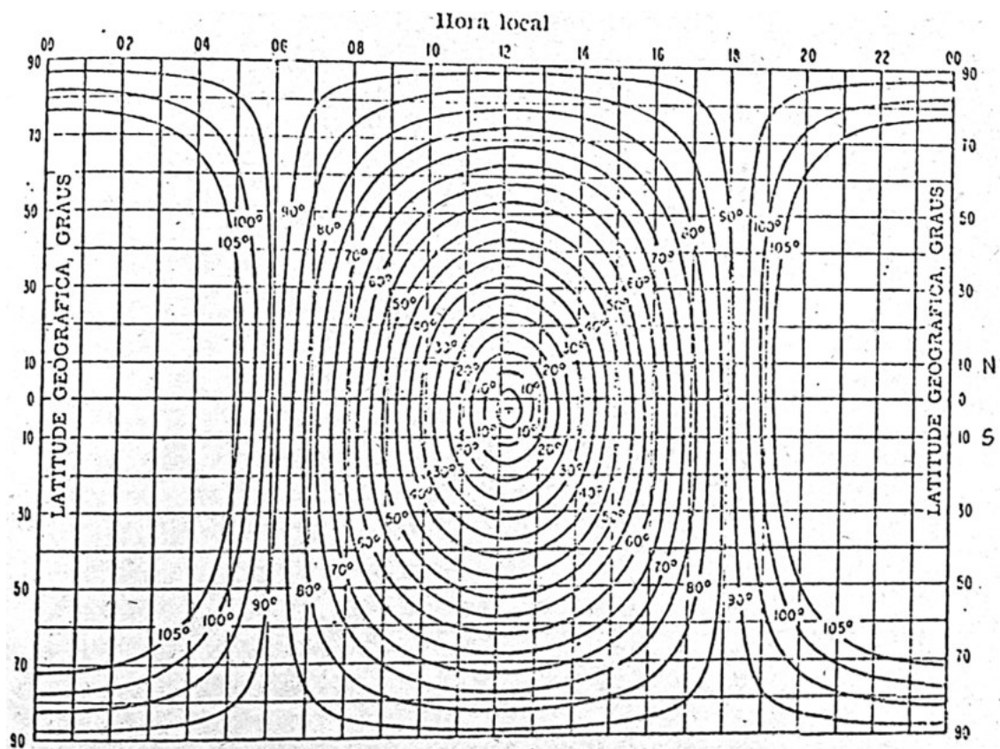
Fig. VI.2 Ângulo zenital do sol, \alpha (março).
