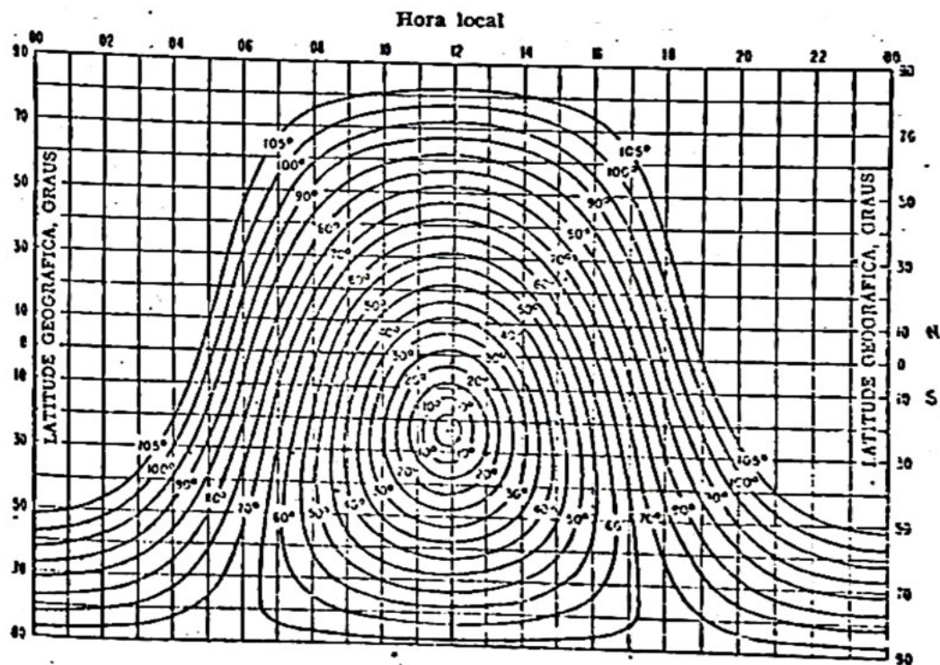
Fig. VI.5 Ângulo zenital do sol, x (dezembro).
