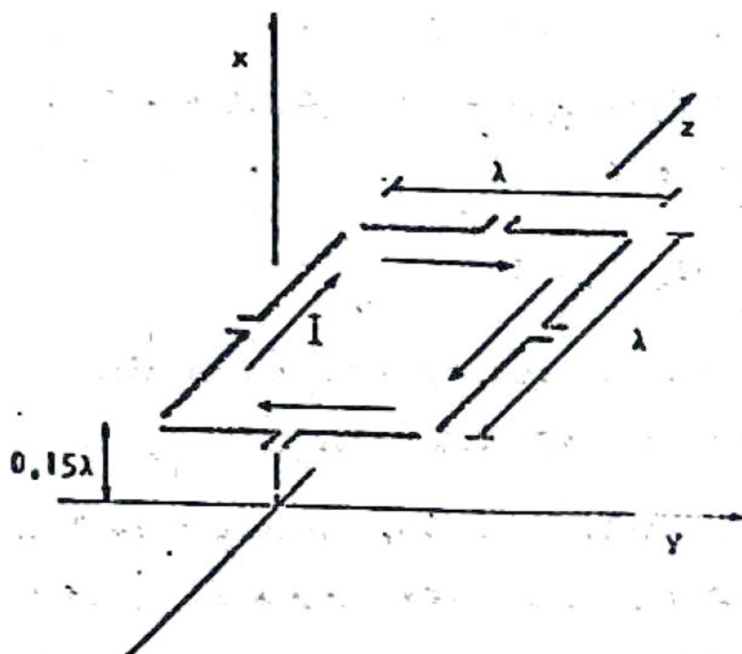
Fig. VII.5 Disposição dos dipolos em uma antena quatro dipolos em quadrado.
