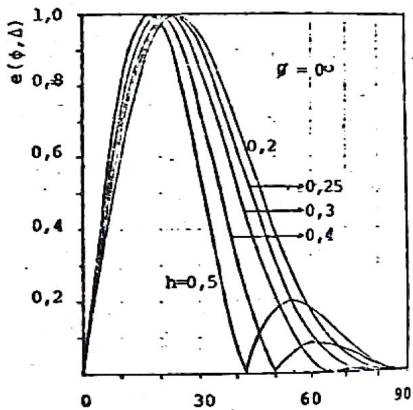
Fig. VII.17 Diagrama Vertical. Antena HR 1/2/\lambda . Refletor Ativo.
