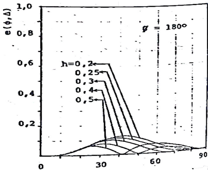
Fig. VII.19 Diagrama Vertical. Antena HR\ 1/2/\lambda . Refletor Ativo.
