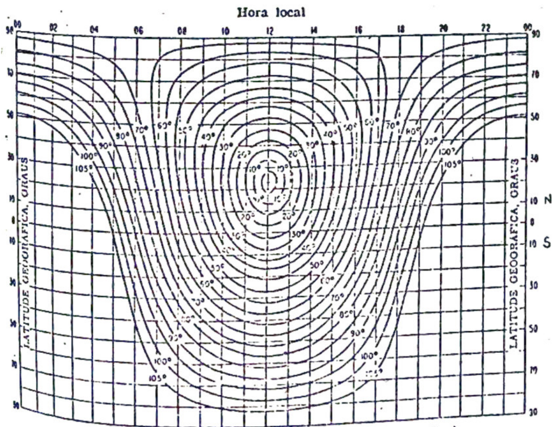
Fig. VI.3 Ângulo zenital do sol, x (junho).
