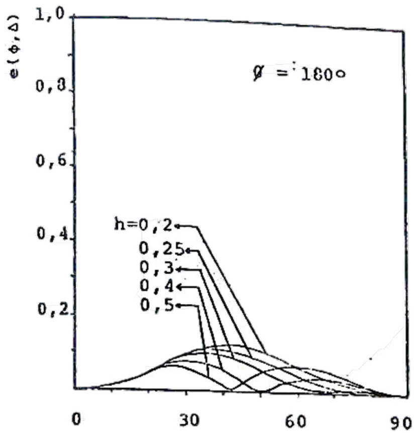
Fig. VII.22 Diagrama Vertical. Antena HR\ 2/2/\frac{h}{\lambda} . Refletor Ativo.
