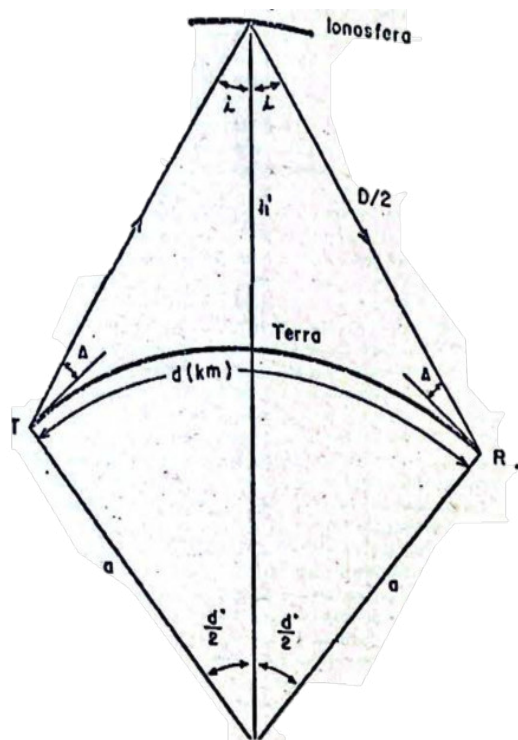
Fig. VI.1 Geometria de Trajeto de um salto via ionosfera.
