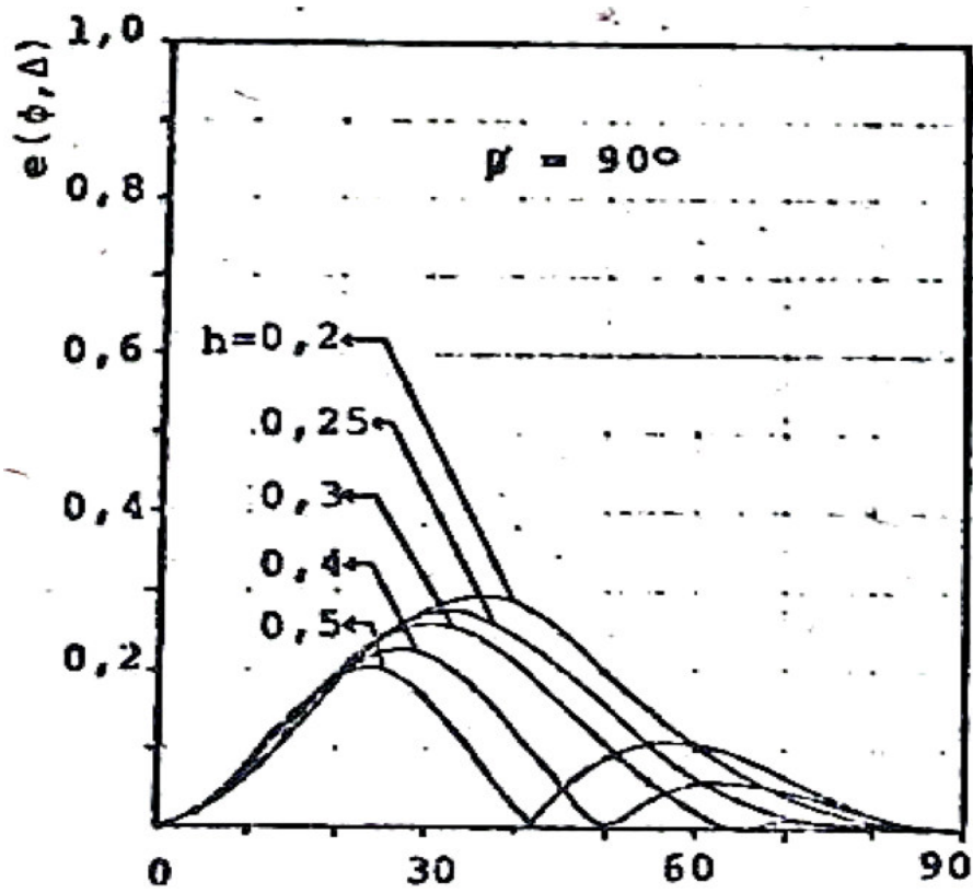
Fig. VII.18 Diagrama Vertical. Antena HR 1/2/\lambda . Refletor Ativo.
