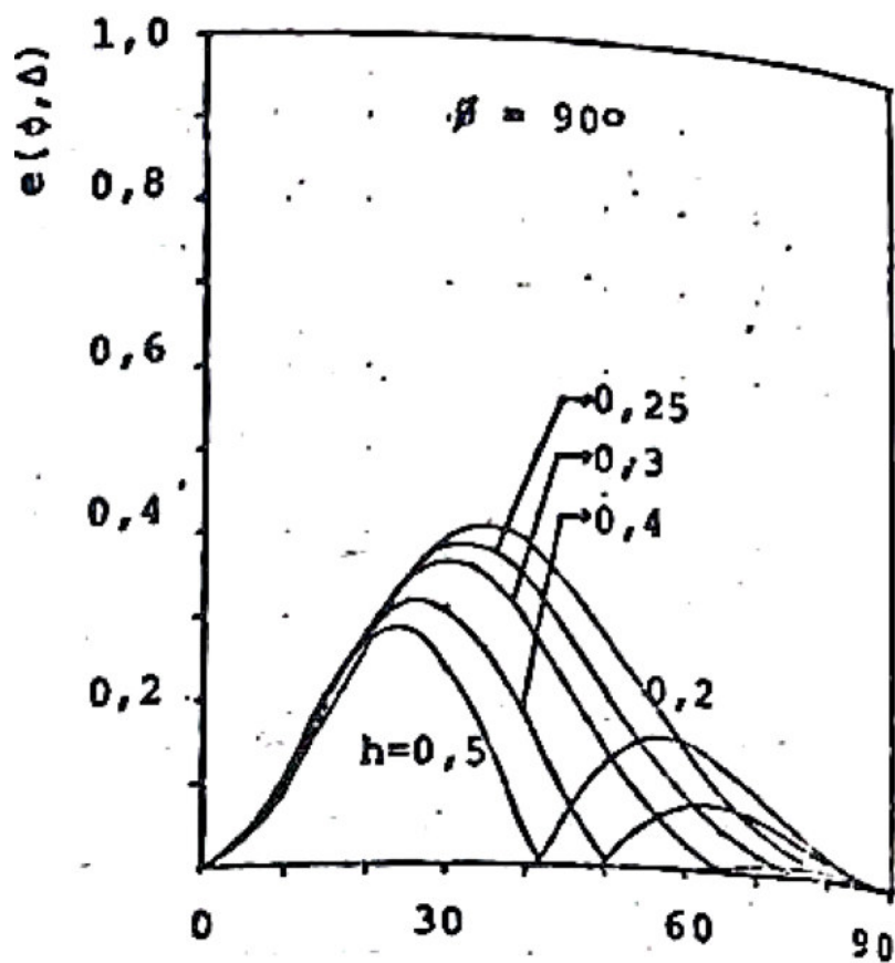
Fig. VII.13 Diagrama Vertical. Antena H \frac{1}{2}\frac{h}{\lambda} .
