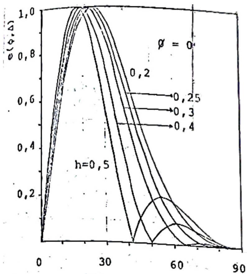
Fig. VII.20 Diagrama Vertical. Antena HR\ 2/2/\lambda . Refletor Ativo.
