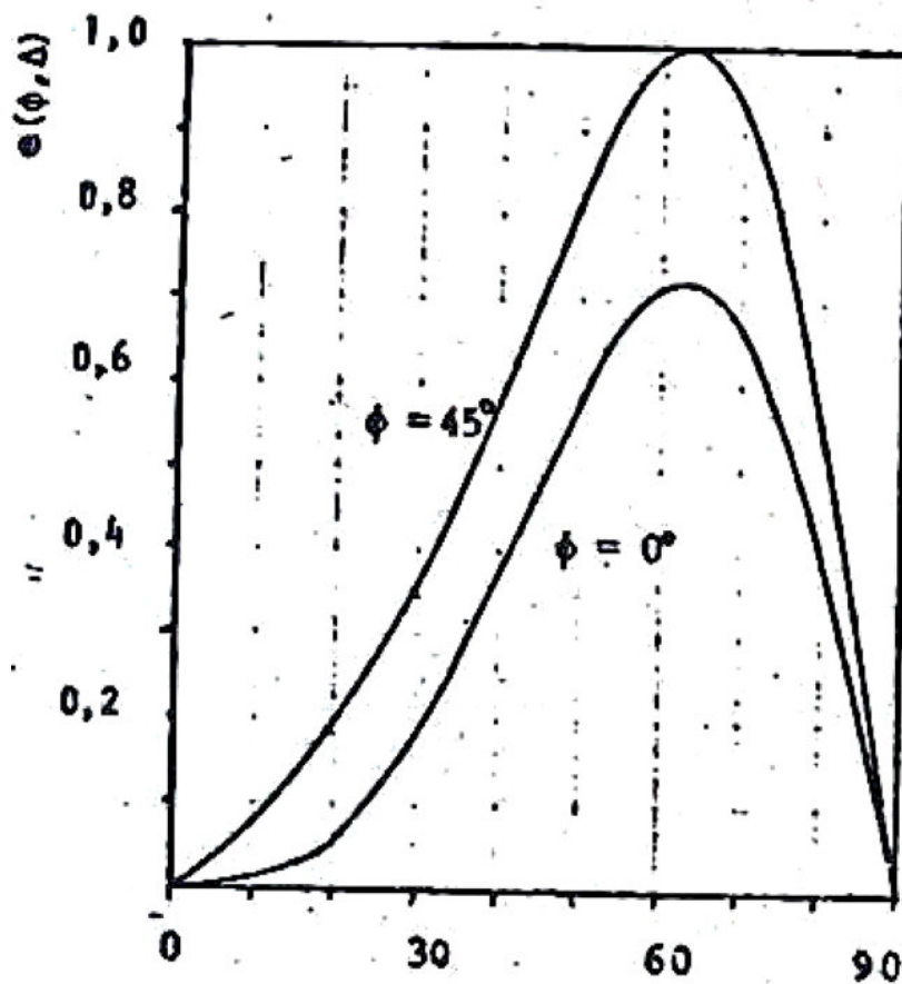
Fig. VII.6 Diagrama Vertical. Antena quatro dipolos em quadrado.
