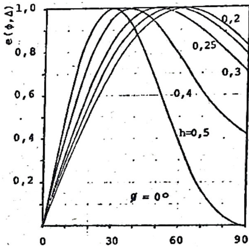
Fig. VII.14 Diagrama Vertical. Antena HR \frac{2}{1}\frac{h}{\lambda} . Refletor Ativo.
