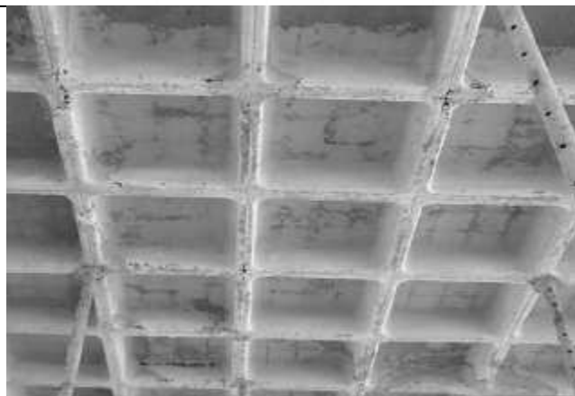
Laje nervurada, presença de segregação de concreto
