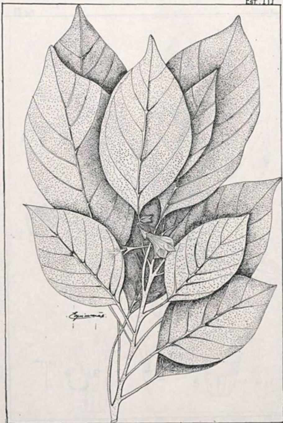
Cordia latifolia Johnston ("Habitus")
