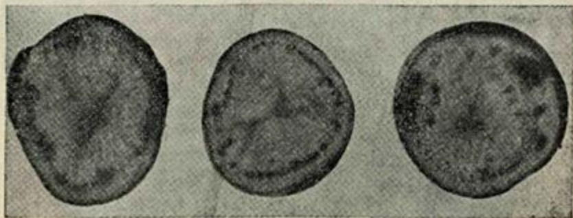
Fig. 2—Tuberculo mostrando o anel escuro.
