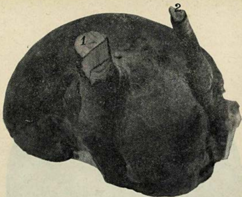
Fig. I—Metade superior da galha. — 1—Ramo principal 2—Ramo secundario fusionado.
