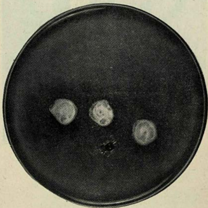
Fig. 4 — Cultura do Bacterium solanaceorum em caixa de Petri.
