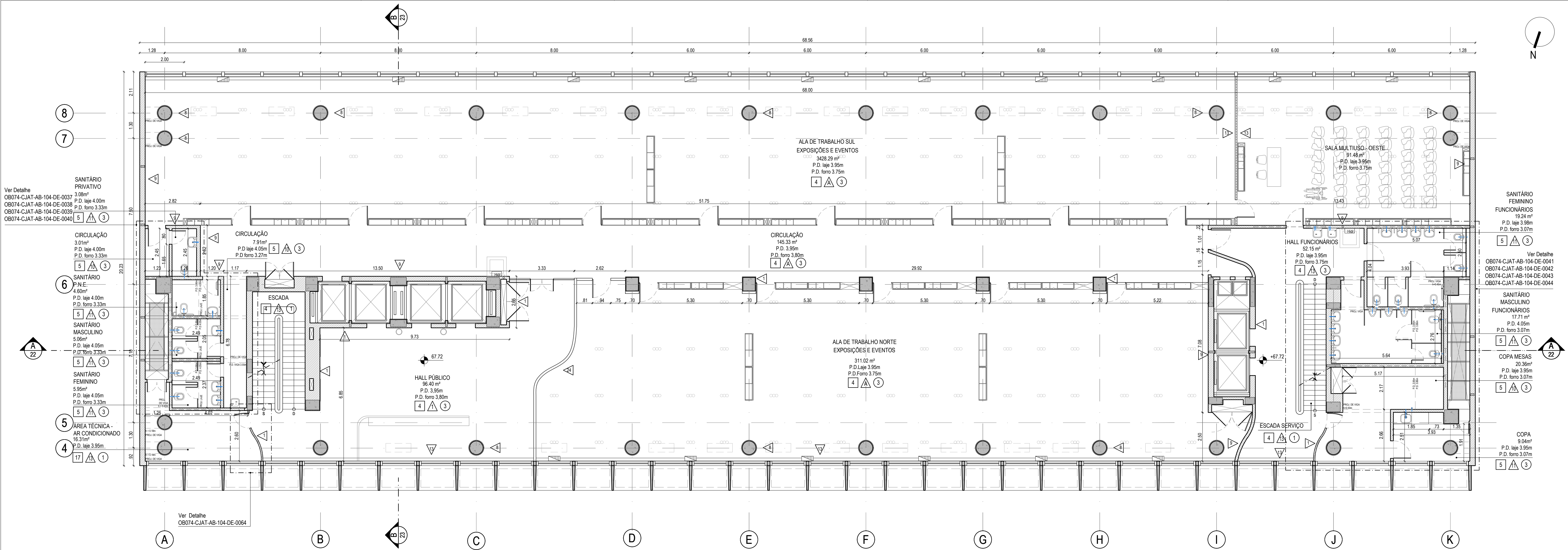
01 PLANTA BAIXA - 15º PAVIMENTO ESC. 1/100
