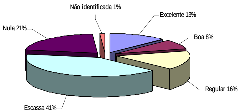
GRÁFICO 8: VISIBILIDADE
