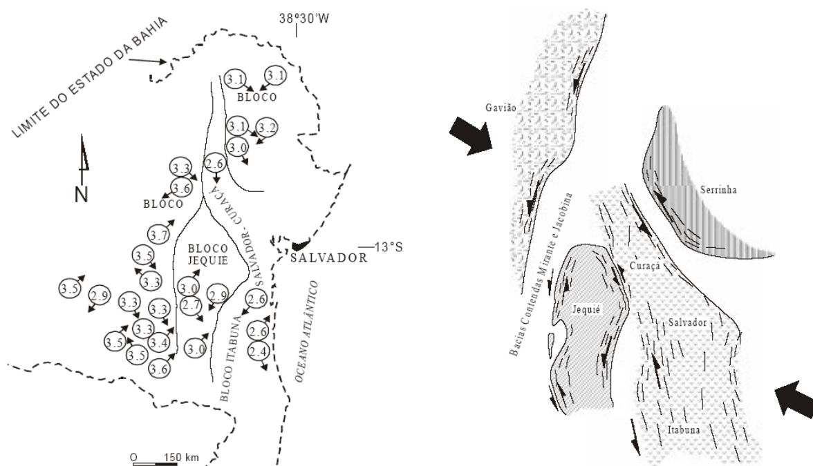
IMAGEM 16: Diferentes unidades estruturais da porção norte do cráton de São Francisco, esquematizando as suas idades geológicas e geotectonismo. Fonte: BARBOSA et al., 2003, p. 9-10.
