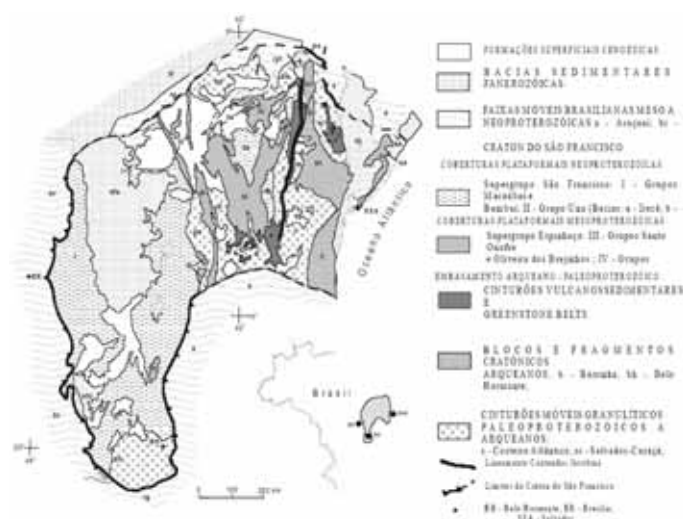
IMAGEM 15: Limites, conformação geológica e compartimentos tectônicos do cráton de São Francisco. Fonte: KOSIN et al., 2003, p. 16.
