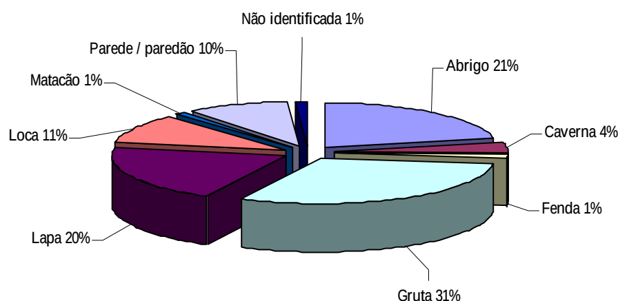
GRÁFICO 6: UNIDADES GEOMORFOLÓGICAS/ARQUEOLÓGICAS
