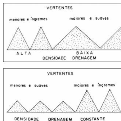
IMAGEM 20: Relação estabelecida entre a densidade da drenagem d'água e a declividade e comprimento das vertentes. Fonte: CHRISTOFOLETTI, 2009 [1980], p. 60.
