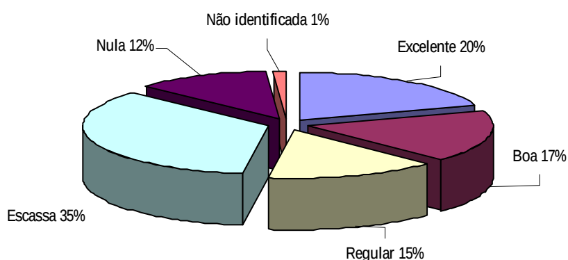
GRÁFICO 7: VISUALIZAÇÃO
