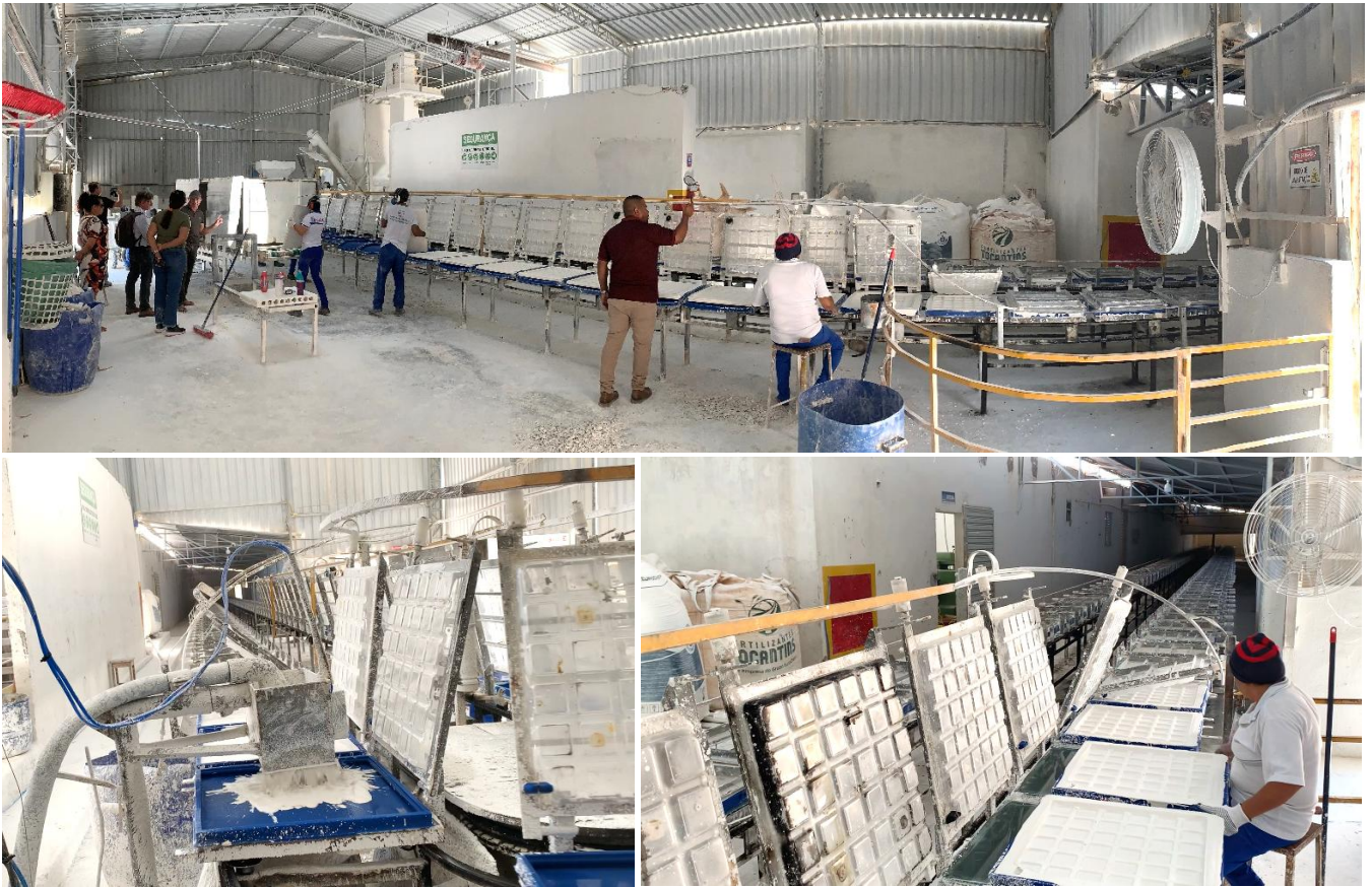
Figura 4. Produção de placas de gesso em “mesas do tipo carrossel”.
