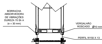
DETALHE 10: SUPORTE DAS CONDENSADORAS SEM ESCALA
