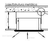
DETALHE 08: FIXAÇÃO DE UNIDADES EVAPORADORAS TIPO CASSETE SEM ESCALA
