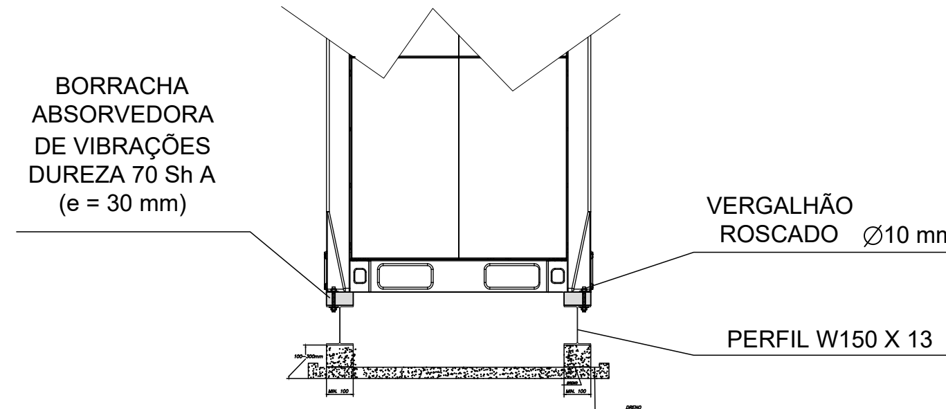
DETALHE 15: SUPORTE DAS CONDESADORAS SEM ESCALA
