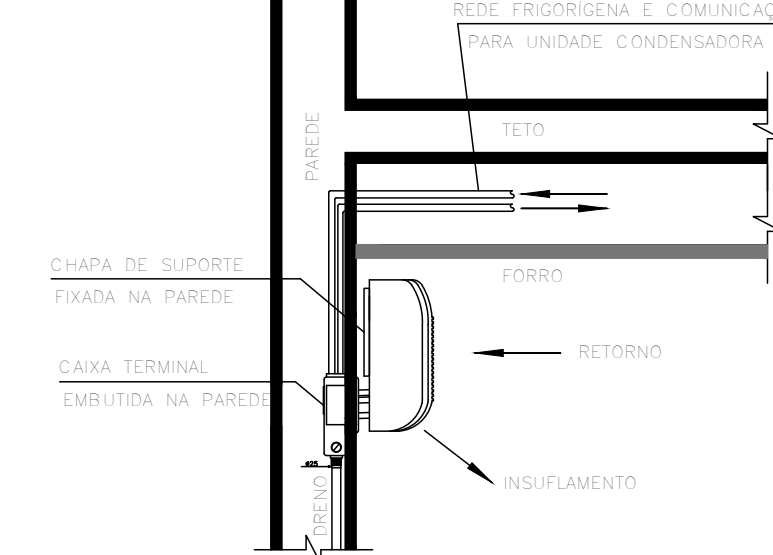
DETALHE 08: FIXAÇÃO DA UNIDADE EVAPORADORA MODELO HI-WALL EM PAREDE SEM ESCALA
