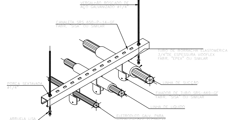
DETALHE 07: ISOLAMENTO TÉRMICO E SUSTENTAÇÃO DAS TUBULAÇÕES FRIGORÍFICAS HORIZONTAIS SEM ESCALA
