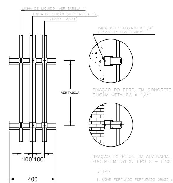
DETALHE 03: SUPORTE VERTICAL EM TUBULAÇÃO FRIGORÍFICA E ELÉTRICA SEM ESCALA
