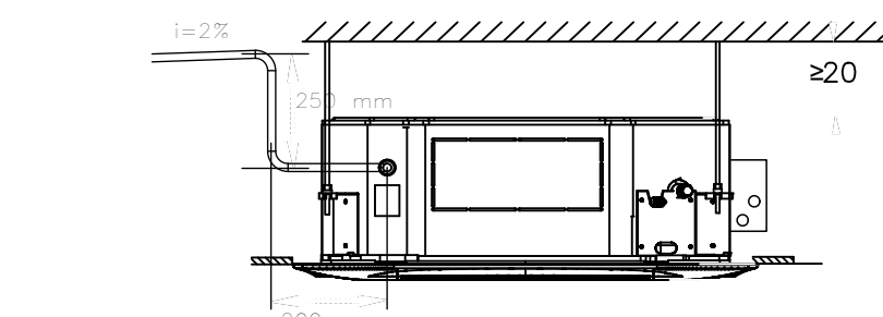
DETALHE 13: DRENO EVAP. CASSETTE SEM ESCALA
