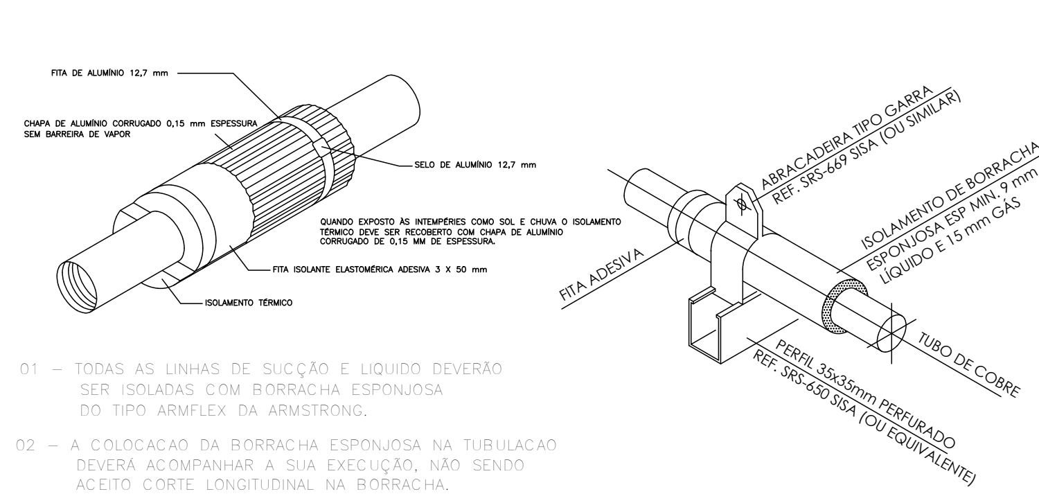
DETALHE 01: ISOLAMENTO EM TUBULAÇÃO FRIGORÍFICA SEM ESCALA
