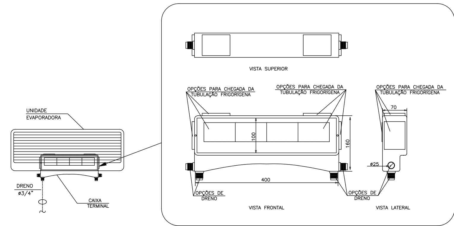
DETALHE 11: CAIXA TERMINAL PLÁSTICA PARA EMBUTIR NA PAREDE SEM ESCALA
