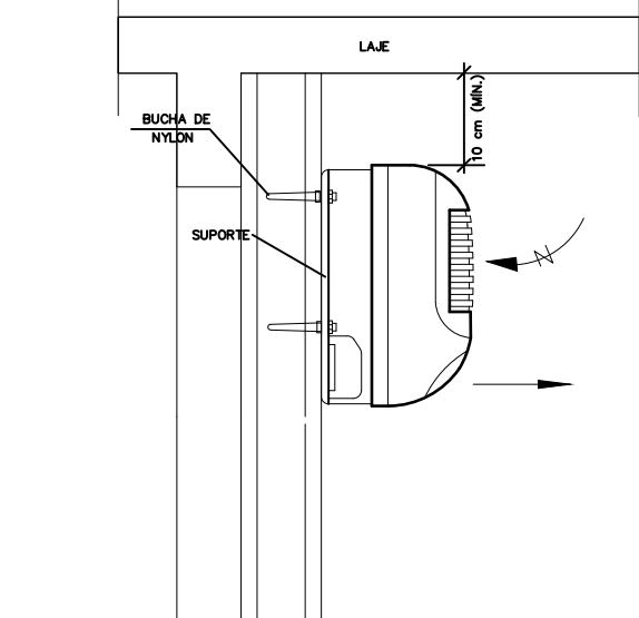
DETALHE 09: INSTALAÇÃO DA EVAPORADORA HI-WALL EM DIVISÓRIA SEM ESCALA
