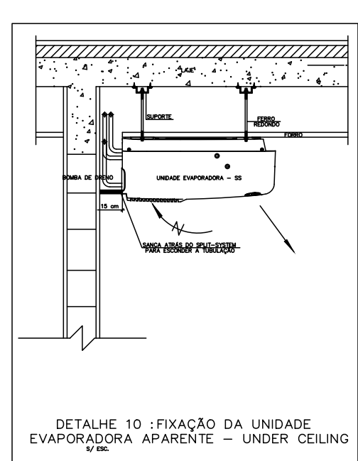
DETALHE 10: FIXAÇÃO DA UNIDADE EVAPORADORA APARENTE - UNDER CEILING SEM ESCALA
