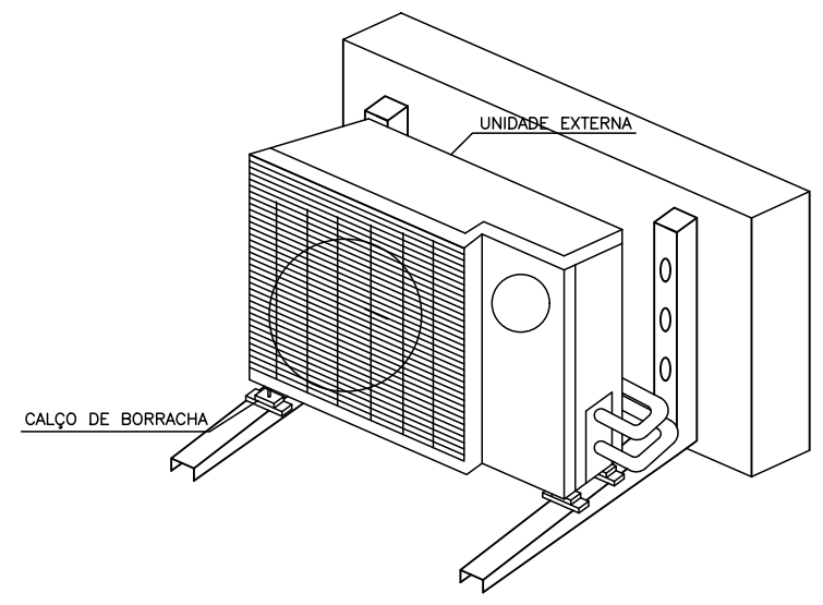
DETALHE 14: SUPORTE DAS CONDESADORAS SEM ESCALA
