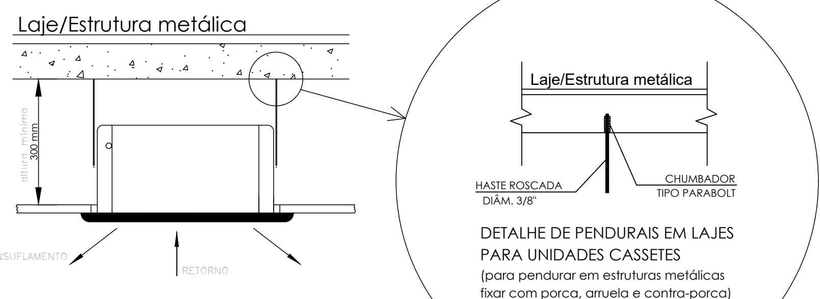
DETALHE 12: FIXAÇÃO DE UNIDADES EVAPORADORAS TIPO CASSETTE SEM ESCALA
