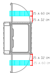
2 VISTA SUPERIOR PLATAFORMAS
