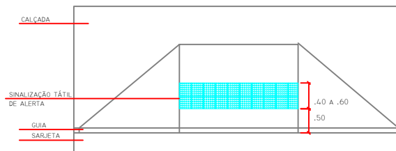
9 VISTA SUPERIOR REBALÇAMENTO DE CALÇADAS
