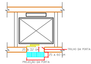
4 VISTA SUPERIOR ELEVADORES
