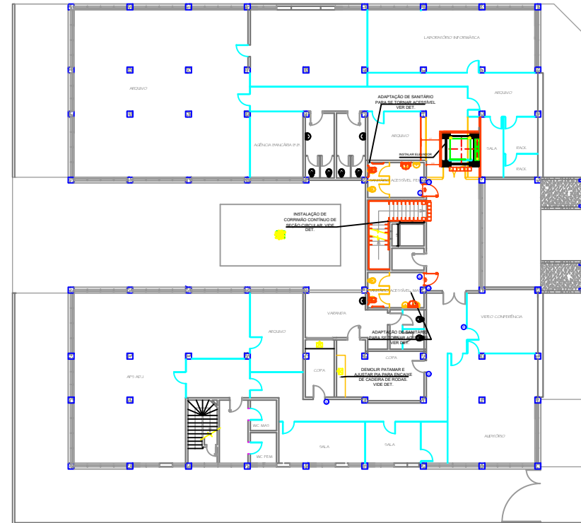
PLANTA BAIXA - Esc.: 1:100 2º ANDAR
