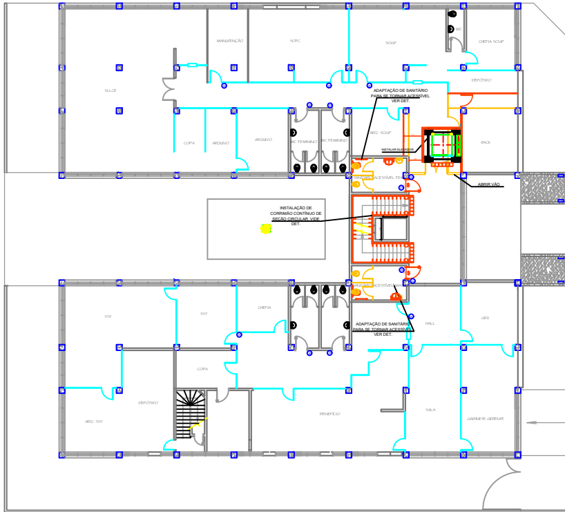
PLANTA BAIXA - Esc.: 1:100 1º ANDAR
