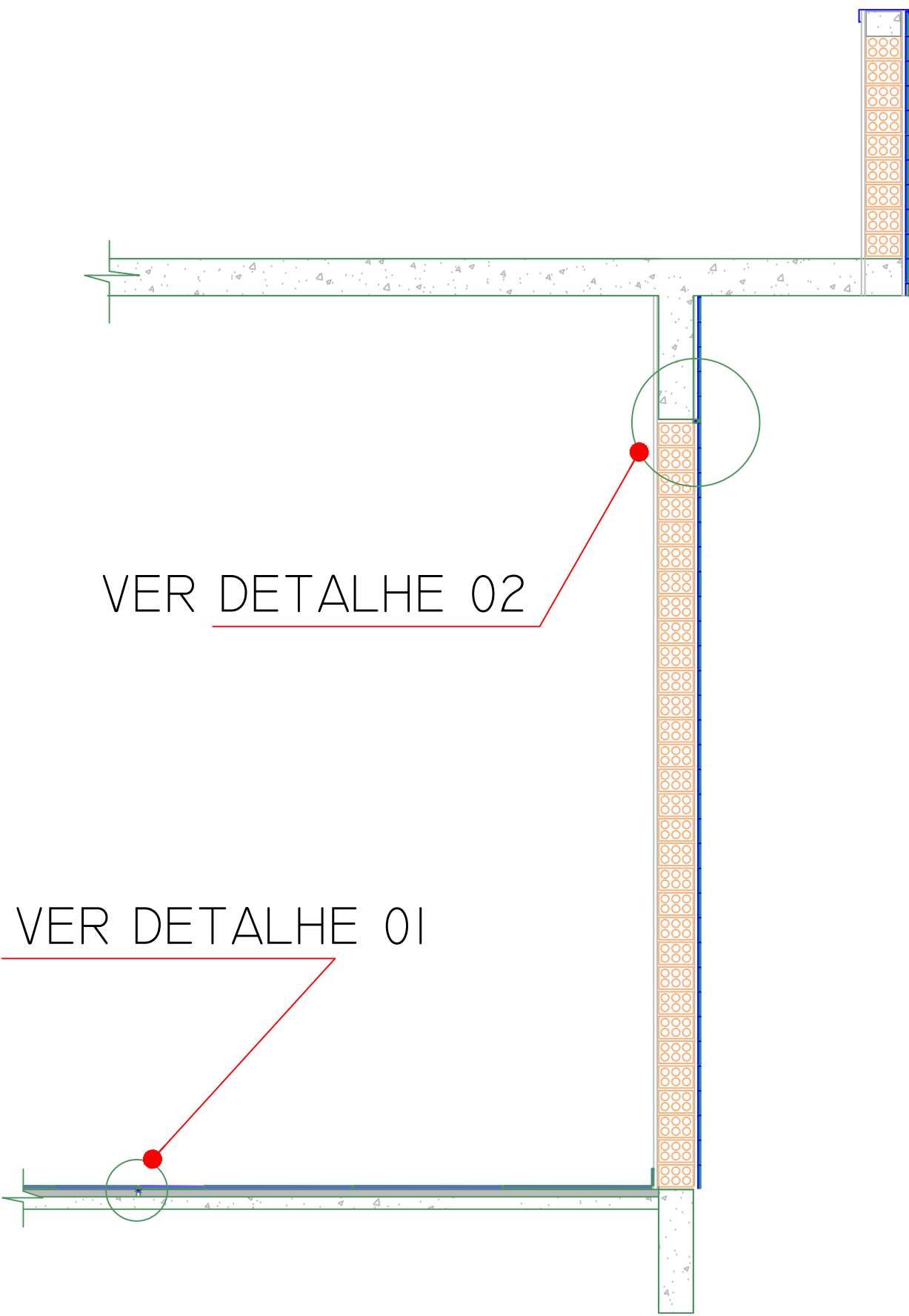
3 CORTE REPRESENTATIVO DE JUNTAS S/ESC.
