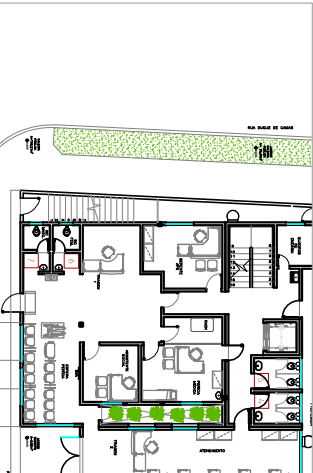
PLANTA BAIXA – PAV. TÉRREO MAPA ÁREAS MOLHADAS ESC.: 1/100
