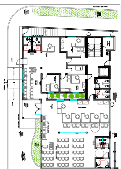
PLANTA BAIXA – PAV. TERREO MAPA ÁREAS MOLHADAS ESC.: 1/100
