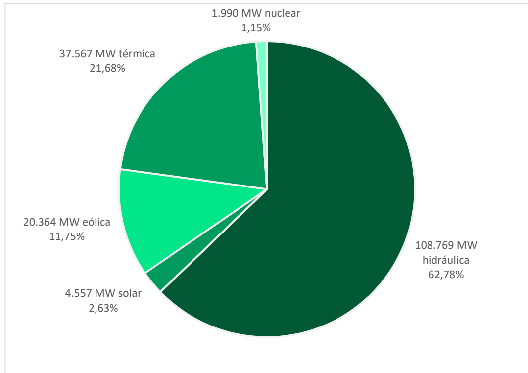
FIGURA 1: ENERGIA NO BRASIL. MATRIZ ELÉTRICA 2021. ADAPTADO DE (ONS) 6 .
