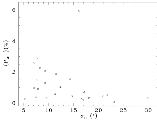
FIGURA 5.11 - Gráfico de dispersão \times polarização média.
