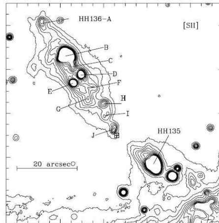
FIGURA 4.1 - HH135/136, um caso onde a direção do jato foi obtida pelos nós de emissão. FONTE: Gredel (2006)
