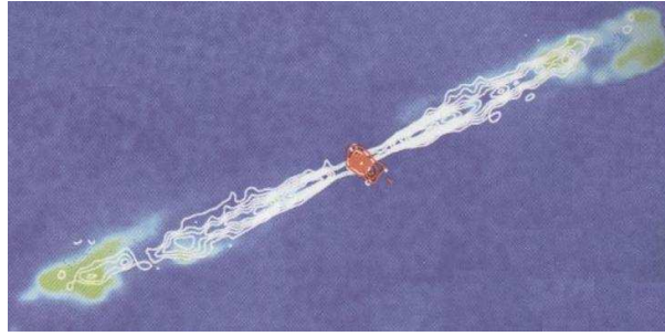
FIGURA 1.9 - Efluxo molecular HH211. Os contornos brancos representam emissão rotacional de CO. Os contornos vermelhos traçam emissão contínua em 1,3mm. A emissão na linha de 2,12 \mu m do H_2 , indicativa de choque, é mostrada em verde. Este objeto poderia ser observado como HH óptico em ambiente menos denso. FONTE: Stahler e Palla (2004)
