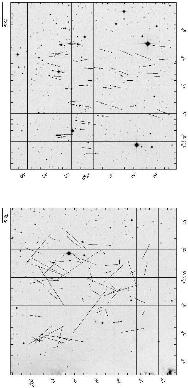
FIGURA A.2 - Distribuição espacial dos vetores de polarização próximos à região de HH19 a 27, 37 e 70. Campo 1 à esquerda e Campo 2 à direita.
