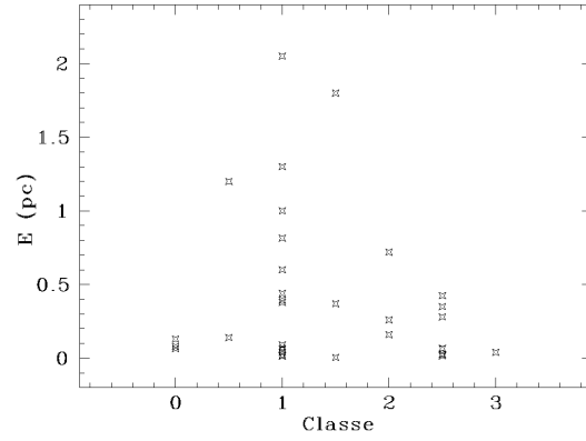
FIGURA 5.5 - Gráfico da classe do OEJ \times extensão do jato.
