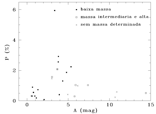
FIGURA 5.12 - Gráfico da polarização média do MI \times extinção do MI com destaque para objetos de diferentes massas.
