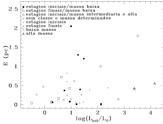
FIGURA 5.4 - Gráfico da L_{bol} do OEJ \times extensão do jato.
