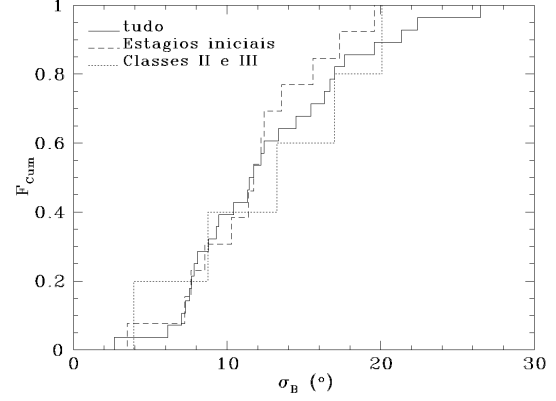
FIGURA 5.8 - Histograma cumulativo das dispersões do CMI para todos os objetos, para os objetos em estágios iniciais de FE e para os objetos de classe II e III.
