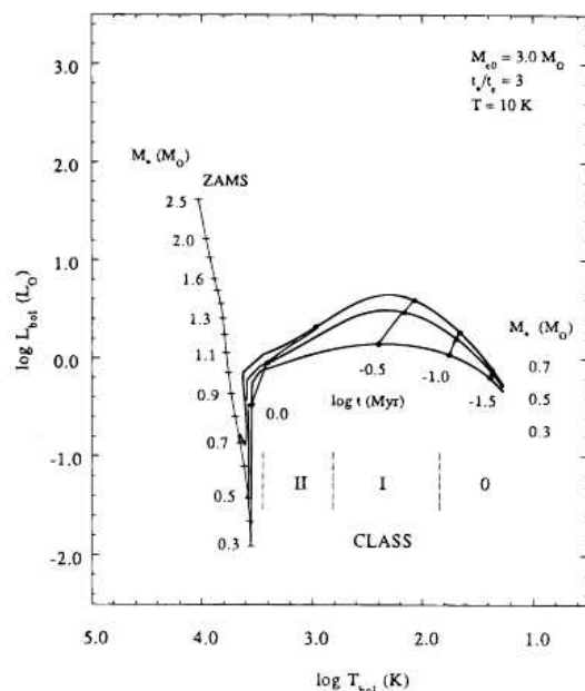
FIGURA 1.4 - Modelo de Myers et al. (1998) para sequência evolutiva de FE.
