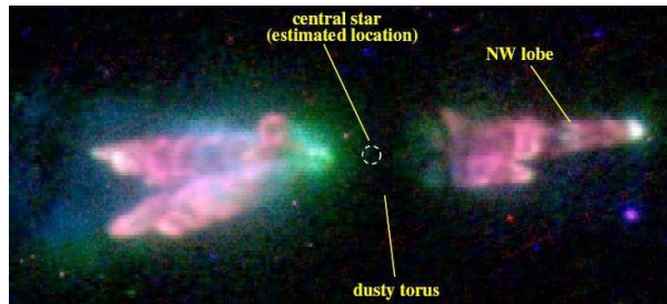
FIGURA 1.10 - Imagem em [OI]\lambda 6300 + H\alpha de CLS618, uma estrela pós-AGB FONTE: Lee et al. (2003)
