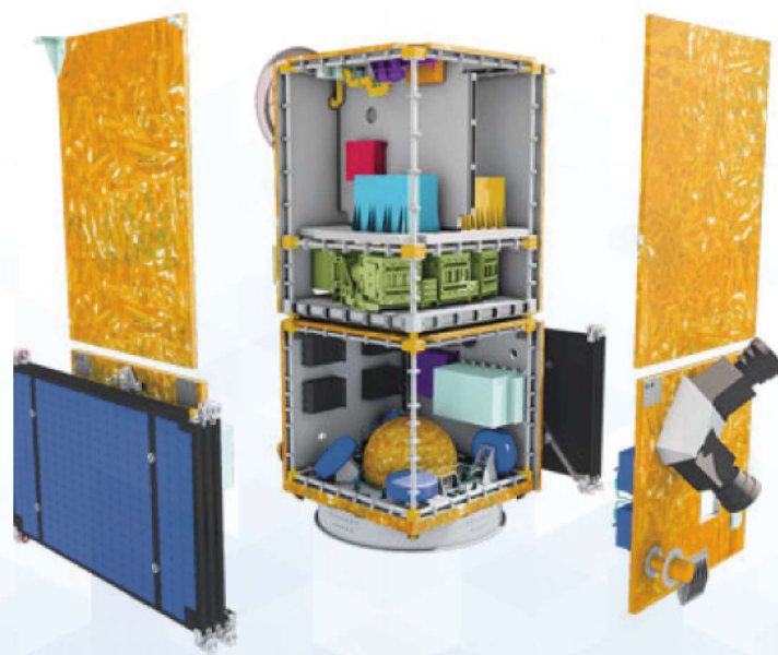
Satélite Amazonia 1 por dentro: PMM acoplada com Módulo de Carga Útil
