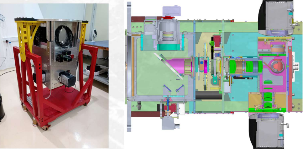
SPARC4 - Polarímetro Simultâneo e Câmera Rápida em 4 bandas dentro do espectro eletromagnético - uma câmera ótica construída no Brasil, para uso da comunidade astronômica brasileira. Será instalada no Laboratório Nacional de Astrofísica, no telescópio de 1,6m. Prevê-se que tenha a sua primeira luz antes do final de 2022.
