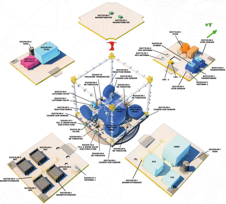
Plataforma Multimissão vista por dentro
