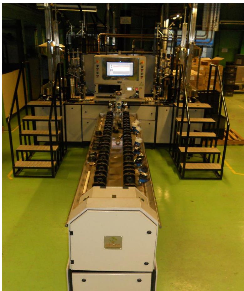
Figura A2 –Bancada de Calibração de Hidrômetros da Empresa - COPASA
