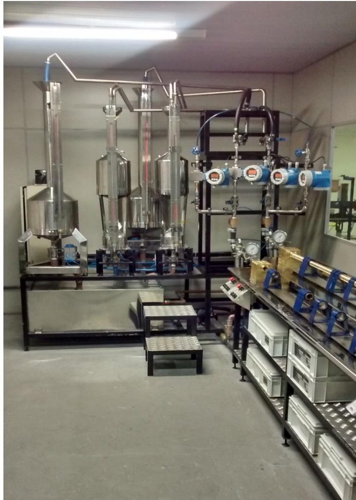
Figura A6 –Bancada de Calibração de Hidrômetros da Empresa - Saga Medição
