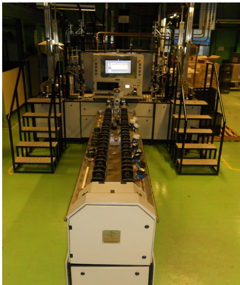
Figura A3 –Bancada de Calibração de Hidrômetros da Empresa – COPASA
