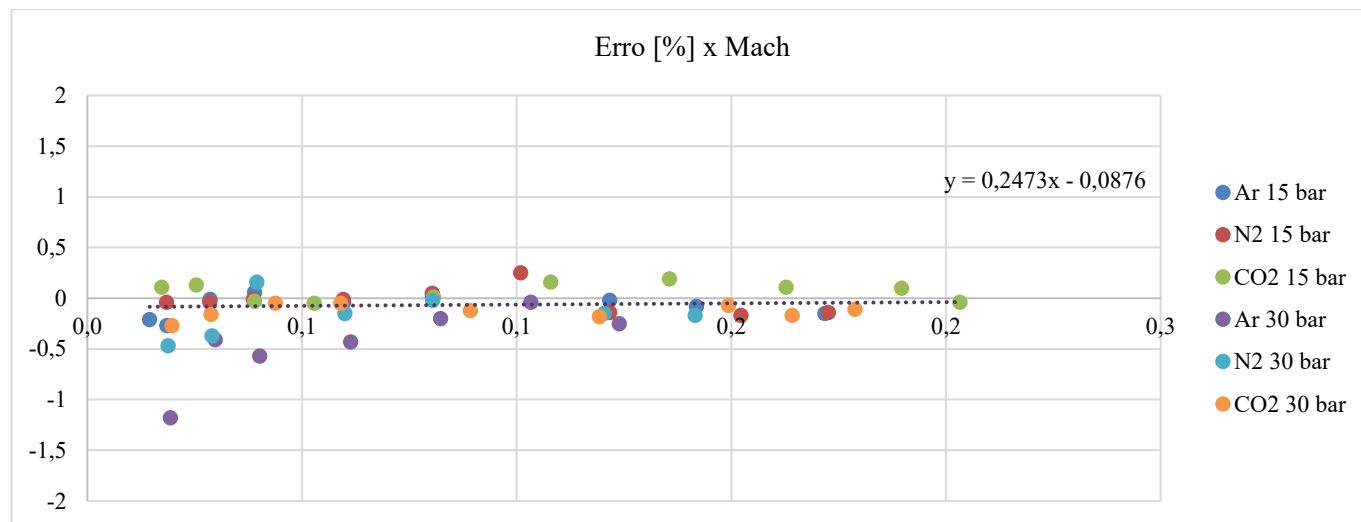
Figura 4 – Análise da influência do número de Mach na medição.
