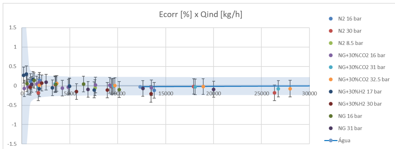
Figura 9 - Resultados de erros de medição corrigidos em função da vazão mássica para ensaios utilizando nitrogênio e misturas de gás natural.
