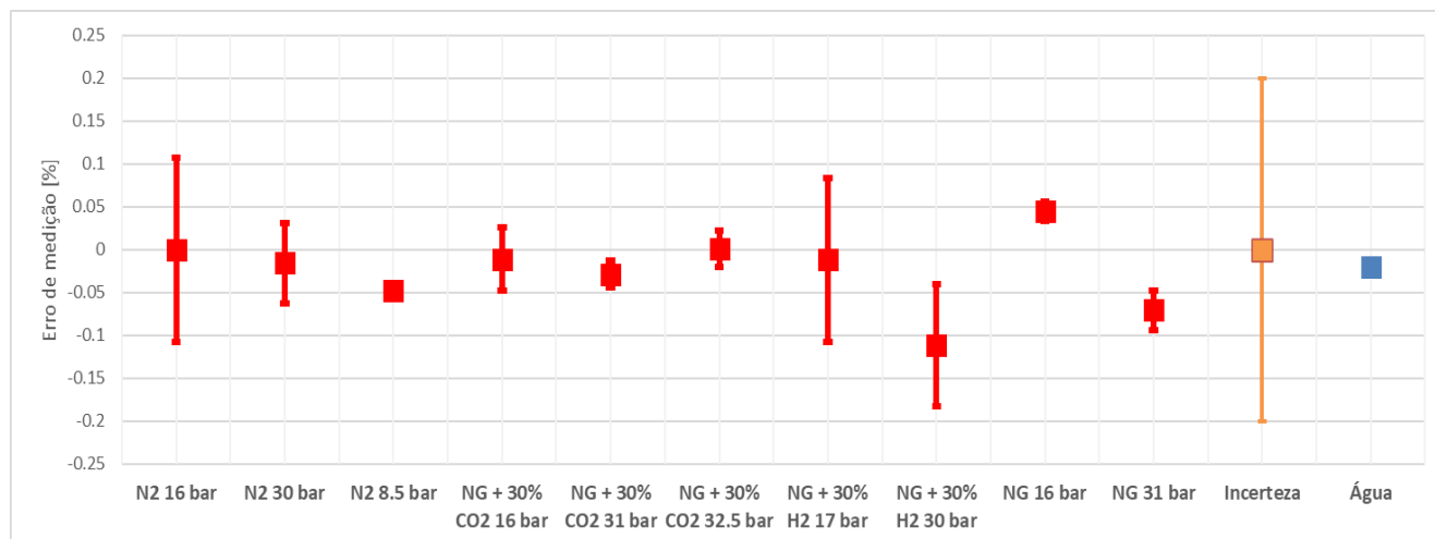
Figura 10 - Comparação das medianas do erro de medição \pm MAD para todos os fluidos ensaiados.
