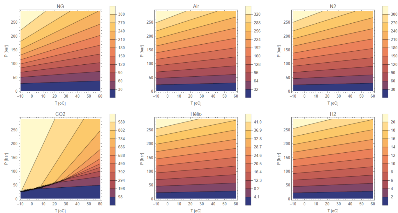
Figura 2 - Densidade [ \text{kg/m}^3 ] em alguns gases, em função da temperatura [ ^{\circ}\text{C} ] e pressão [bar]
