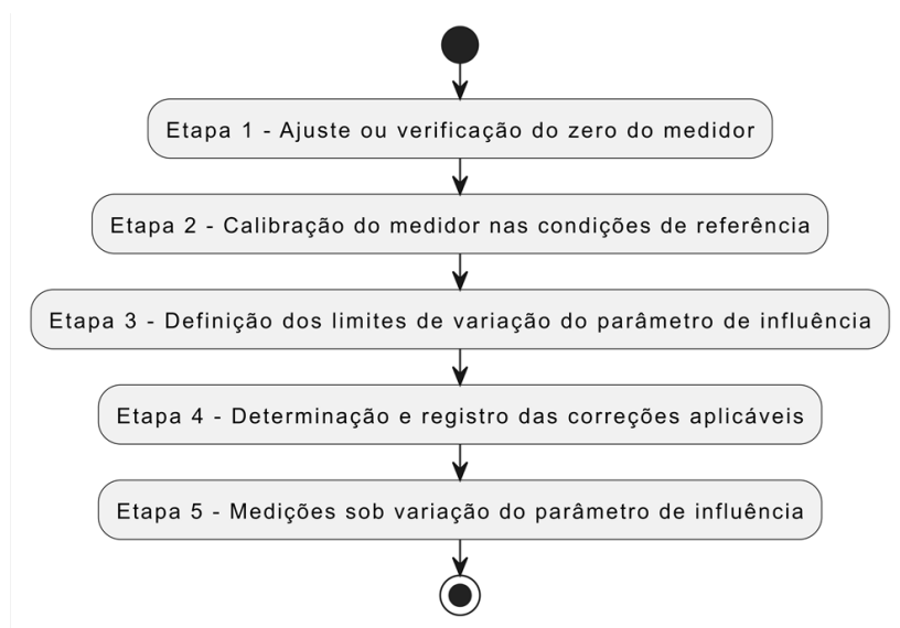
Figura 2 - Procedimento para caracterização do medidor.
