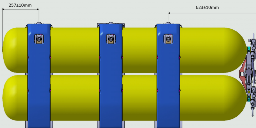
Figura 5: Posicionamento das cintas para cilindros de 118L
