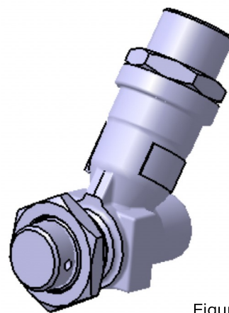
Figura 9: Válvula de abastecimento tipo NBR
