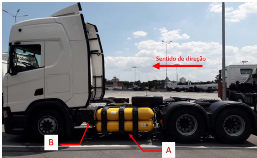
Figura 17: Vista do lado esquerdo do veículo 6x2
