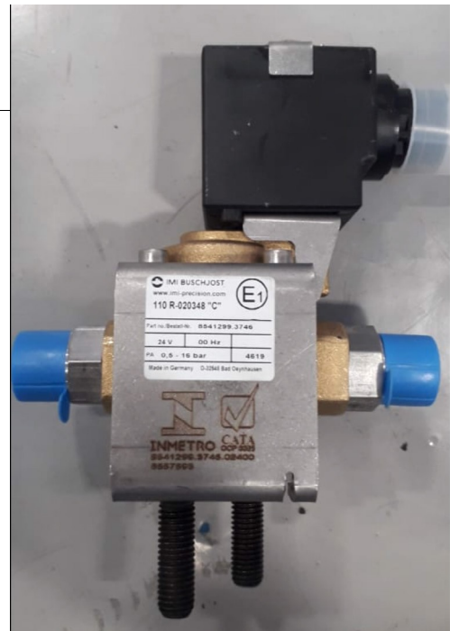
Figura 16: Válvula solenoide de baixa pressão
