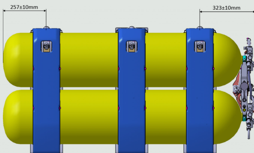
Figura 4: Posicionamento das cintas para cilindros de 95L
