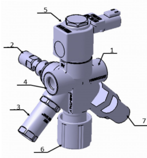
Figura 8: Válvula do cilindro
