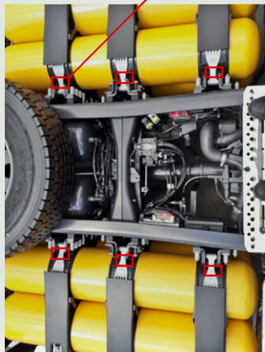
Figura 20: Vista superior, posição das marcações de certificação dos suportes
