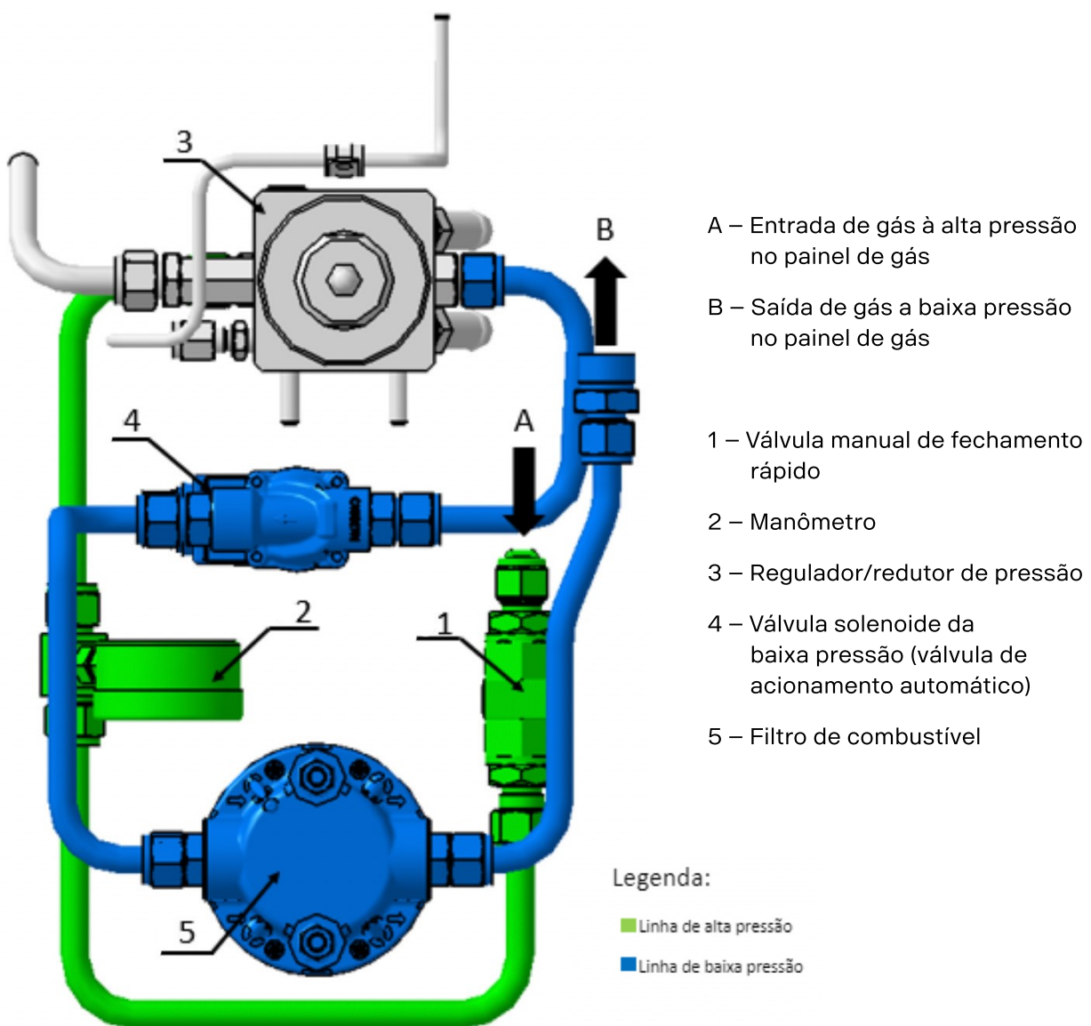
Figura 12: Arquitetura do painel de gás
