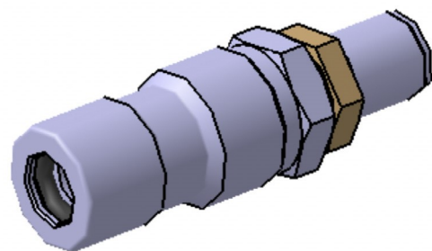
Figura 10: Válvula abastecimento tipo NGV2
