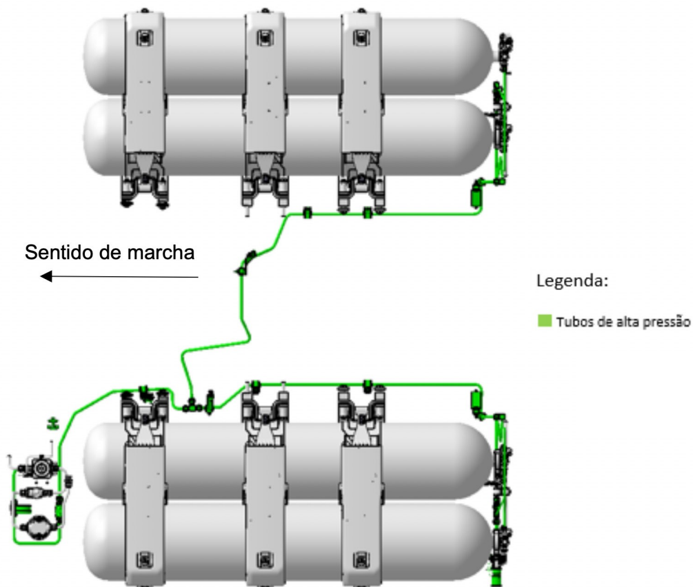
Figura 6: Posicionamento das cintas para cilindros de 118L
