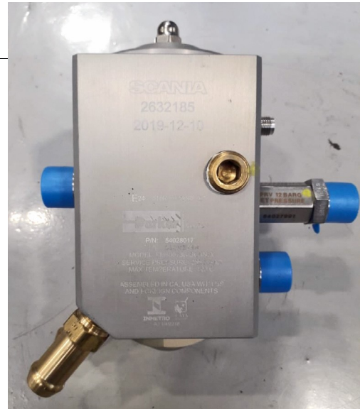
Figura 15: Regulador/redutor de pressão
