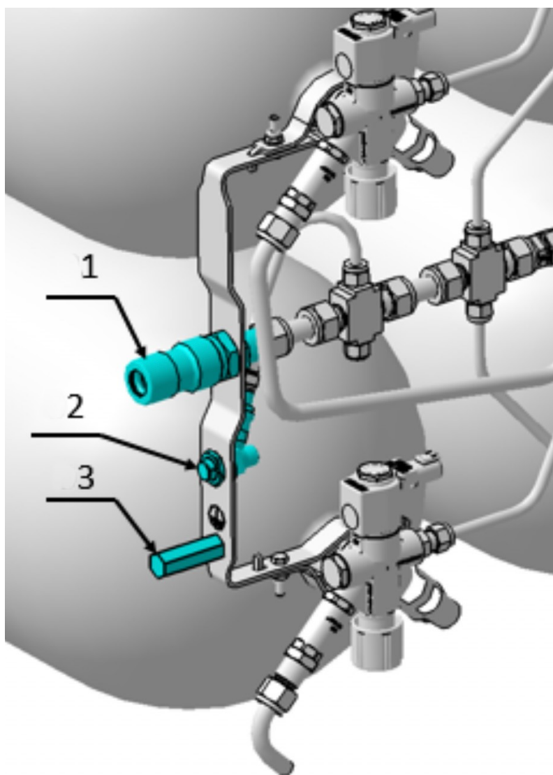
Figura 11: Localização das válvulas de abastecimento
