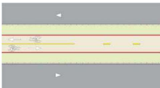
Sinalização Horizontal para Ciclovia/Ciclofaixa - Padrão I
