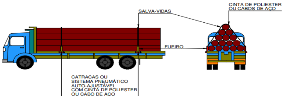
Figura 2 - Carroceria para transporte de toras longitudinal com arrumação piramidal (triangular)
