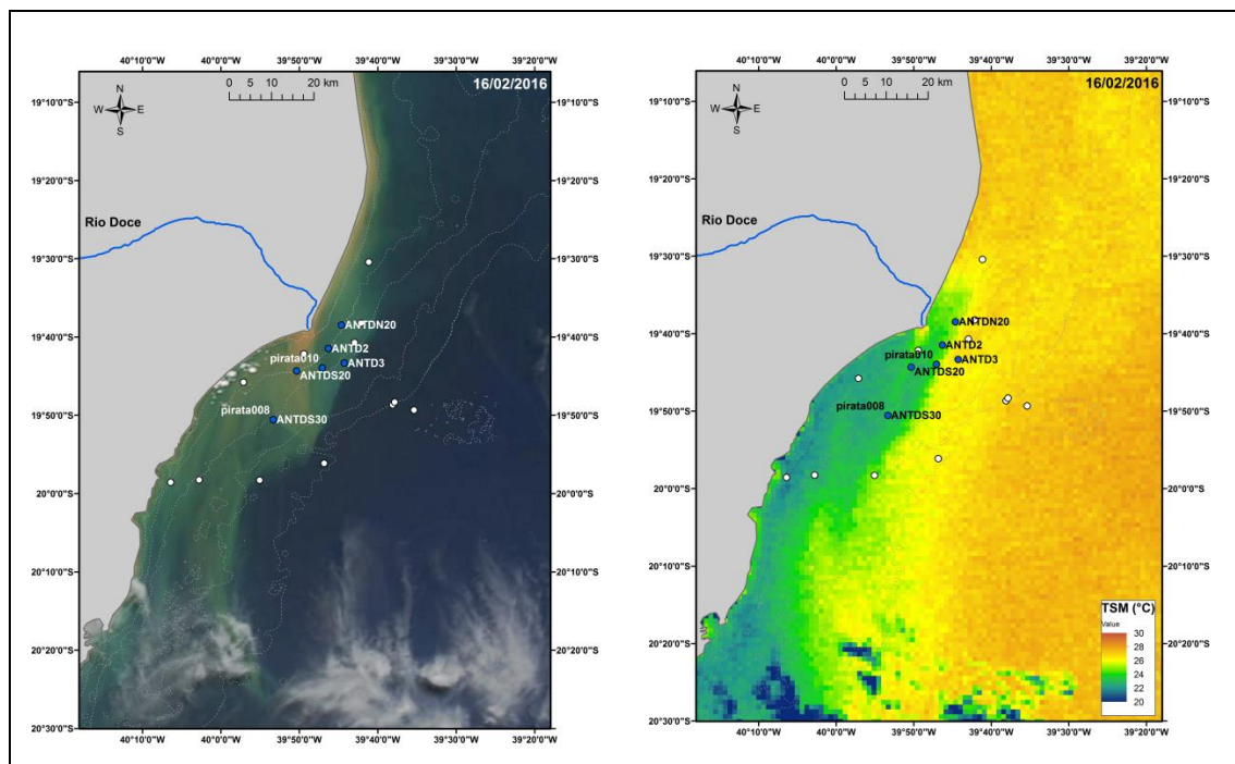
Figura 16: Imagens de cor verdadeira (esquerda – MODIS/Aqua) e temperatura da superfície do mar (direita – MODIS/Aqua). Os pontos brancos identificam as coletas realizadas durante a campanha a bordo do Noc. Antares e os pontos em azul marcam as coletas realizadas no mesmo dia em que a imagem foi obtida.
