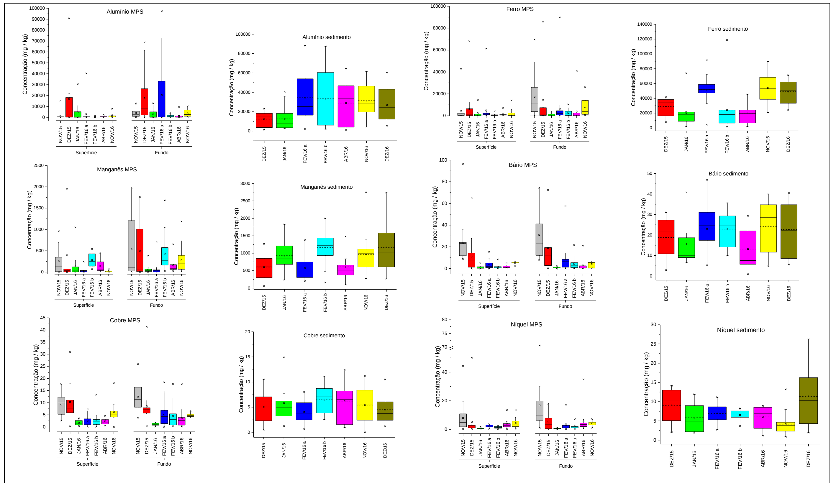
Figura 20: Concentra  o (mg / kg) no material particulado em suspens o e sedimento superficial de Al m nio (Al), Mangan s (Mn), Ferro (Fe), B rio (Ba), Cobre (Cu) e N quel (Ni) durante a chegada da lama de rejeitos na regi o costeira adjacente da foz do Rio Doce.
