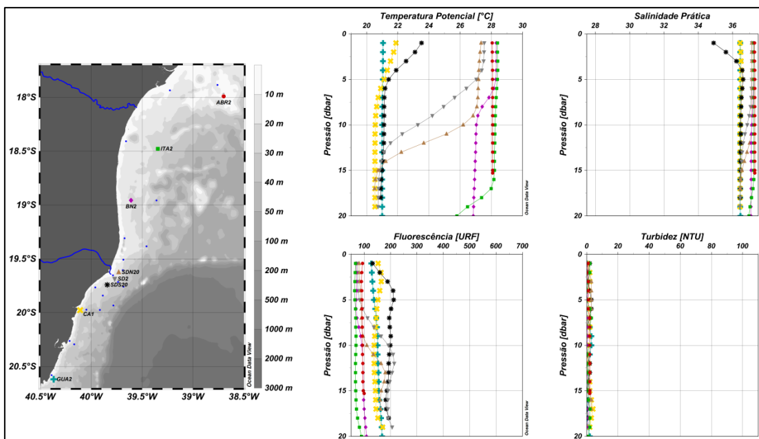
Figura 24: Perfis verticais de Temperatura Potencial ( ^{\circ}\text{C} ), Salinidade Prática, Fluorescência (URF) e Turbidez (NTU) das estações oceanográficas realizadas ao longo do arco de 20 m de profundidade durante a campanha a bordo do Noc. Soloncy Moura.
