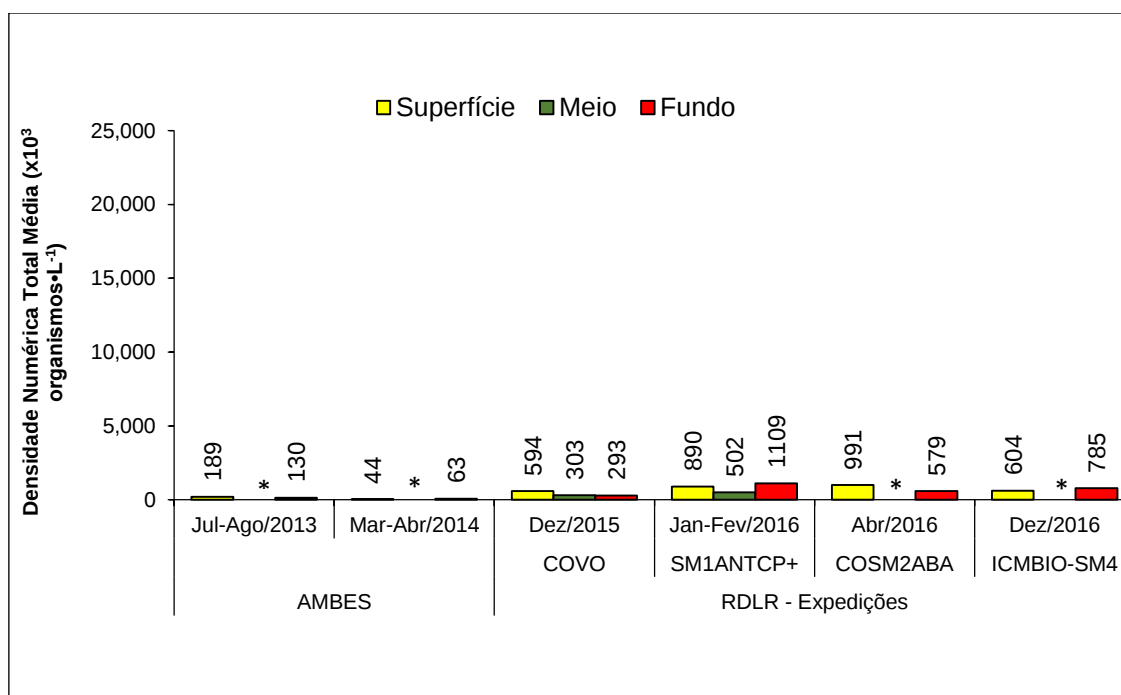
Figura 22: Dados pretéritos defronte à foz do rio Doce obtidos no projeto AMBES e média da densidade numérica do fitoplâncton total ( \times 10^3 \text{ organismos}\cdot\text{L}^{-1} ) de todas as Expedições Oceanográficas realizadas ao longo do monitoramento do Projeto Rio Doce Lama de Rejeito (RDRL).
