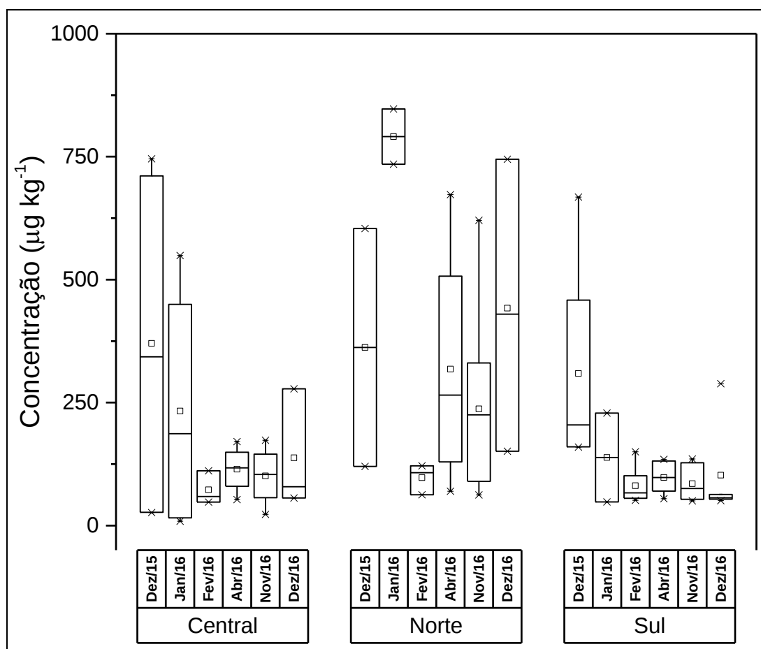
Figura 45 - Distribuição dos valores de mínima, máxima, média e mediana das concentrações de HPA total nas campanhas de amostragem na foz do rio Doce e plataforma adjacente.
