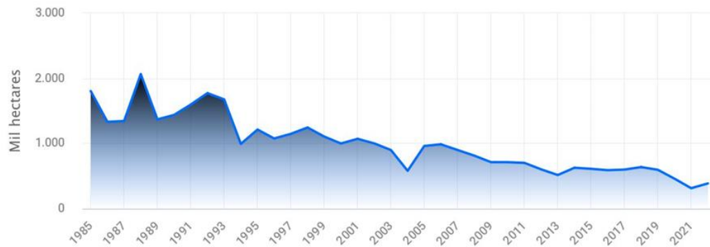
Série temporal da superfície d'água - Pantanal
