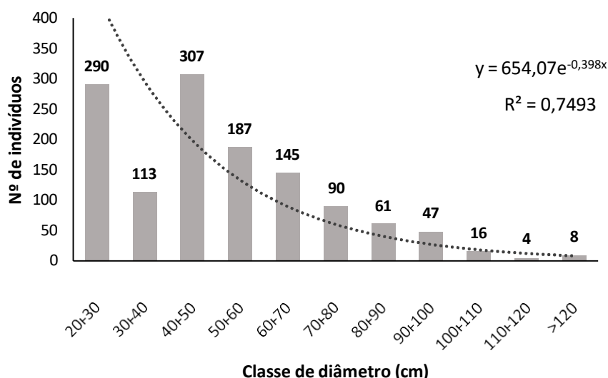
Figura 5 - Distribuição diamétrica dos indivíduos
