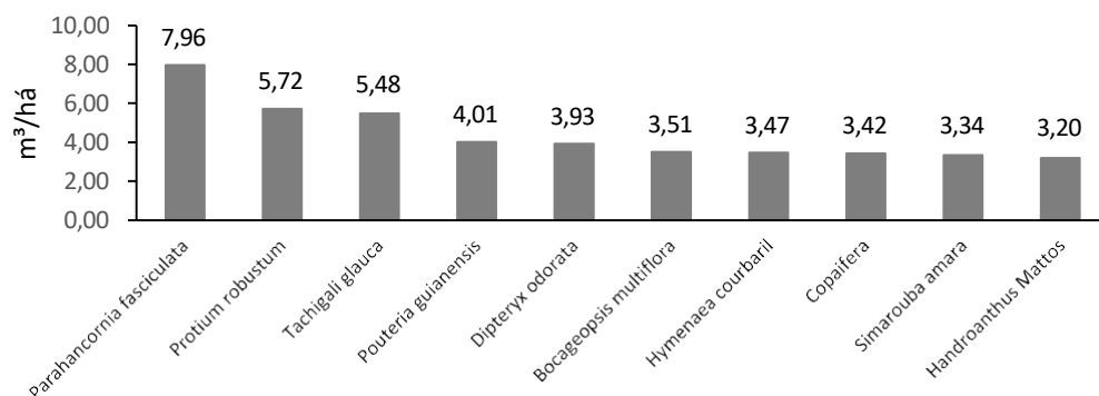
Figura 7 - Volume fator de forma (0,68) ( \text{m}^3/\text{ha} )
