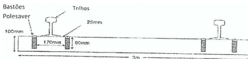
Figura 1. Aplicação de Polesaver Rods em dormentes.
