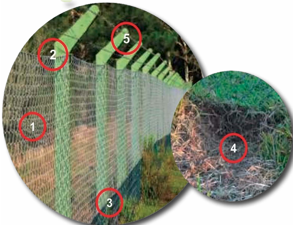
Figura 10 – Cerca para exclusão em granjas de suínos (Fonte: Bordin, Kramer, Silva, 2013).
