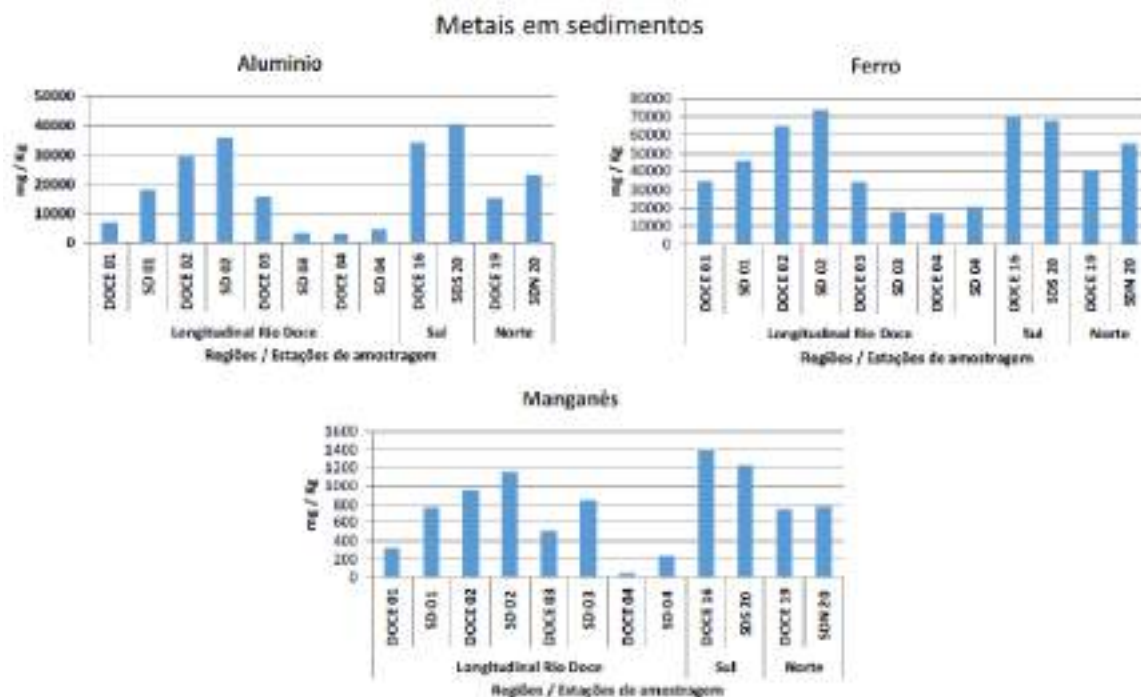
Figura 11 - Gráfico das concentrações de alumínio, ferro e manganês nos sedimentos superficiais da foz do Rio Doce nas estações de amostragem da primeira campanha (Doce) e da segunda campanha (SD) do monitoramento marinho. Fonte: Neto et al (2016)
