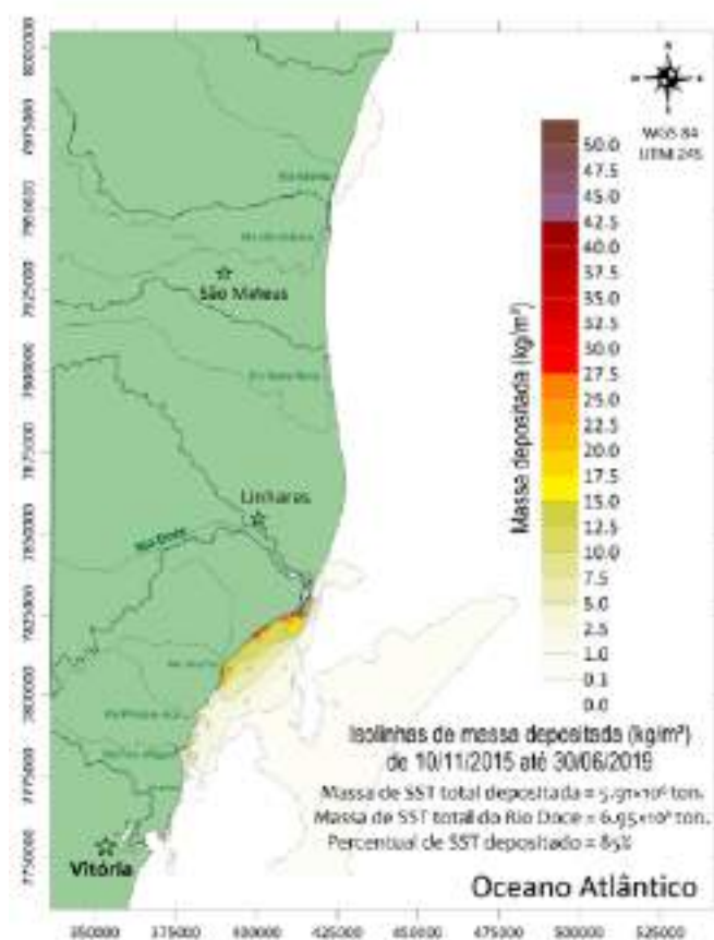
Figura 2 - Mapa de isolinhas de massa depositada de lama inconsolidada oriunda da carga de Sólido Suspenso Total (SST) do Rio Doce, entre 10/11/2015 e 30/06/2019. A massa total de SST vinda pelo Rio Doce chegou a 6.95 milhões de toneladas, das quais
