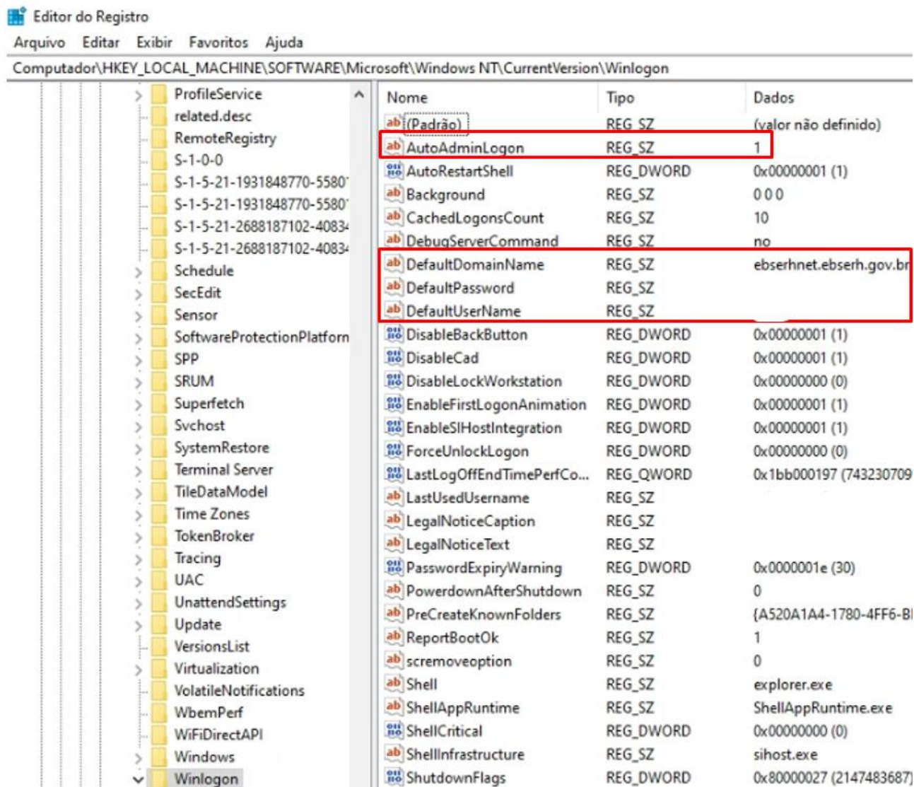
Figura 1: Tela de configurações de parâmetros do login Windows
