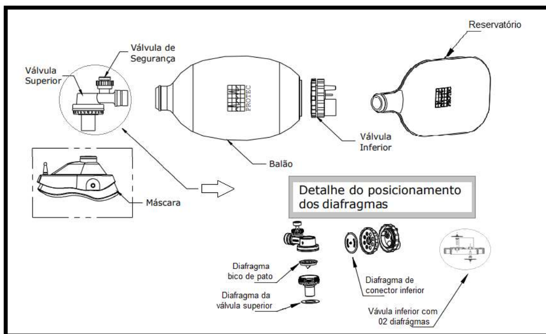
Figura 01 –Reanimador manual e seus principais componentes
