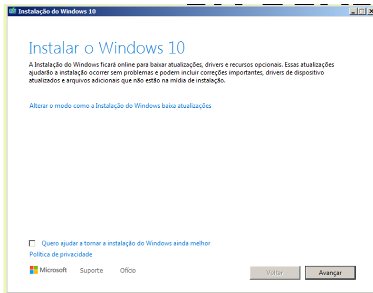
Figura 4 – Iniciando instalação.
