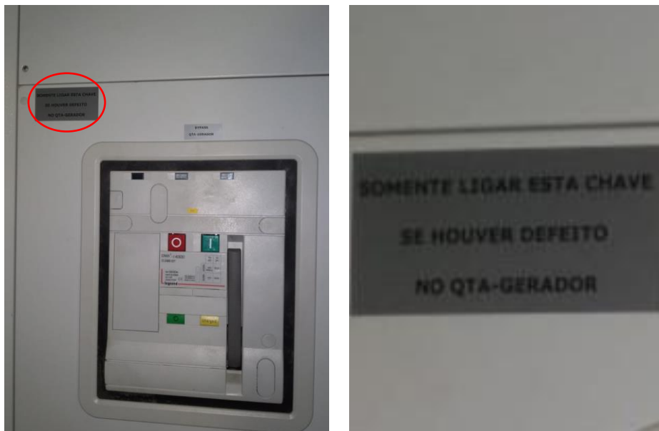
Figura 16 – Exemplos do sistema de by-pass do grupo gerador e indicação do aviso
