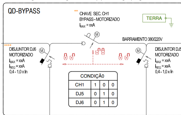
Figura 14 – Diagrama do by-pass do grupo gerador
