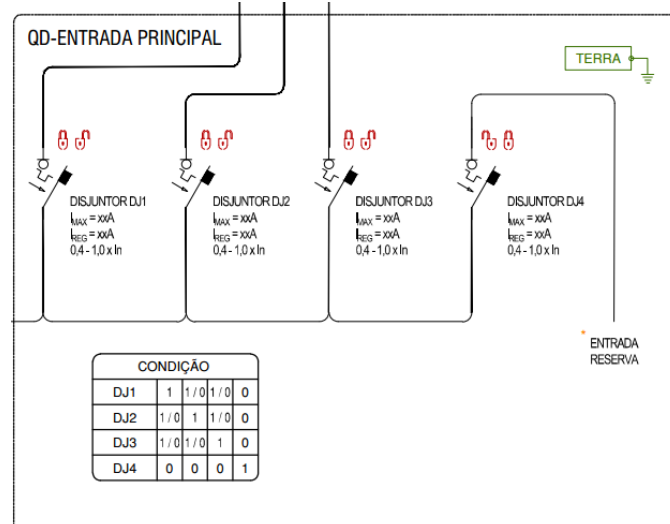
Figura 15 – Diagrama do by-pass do grupo gerador
