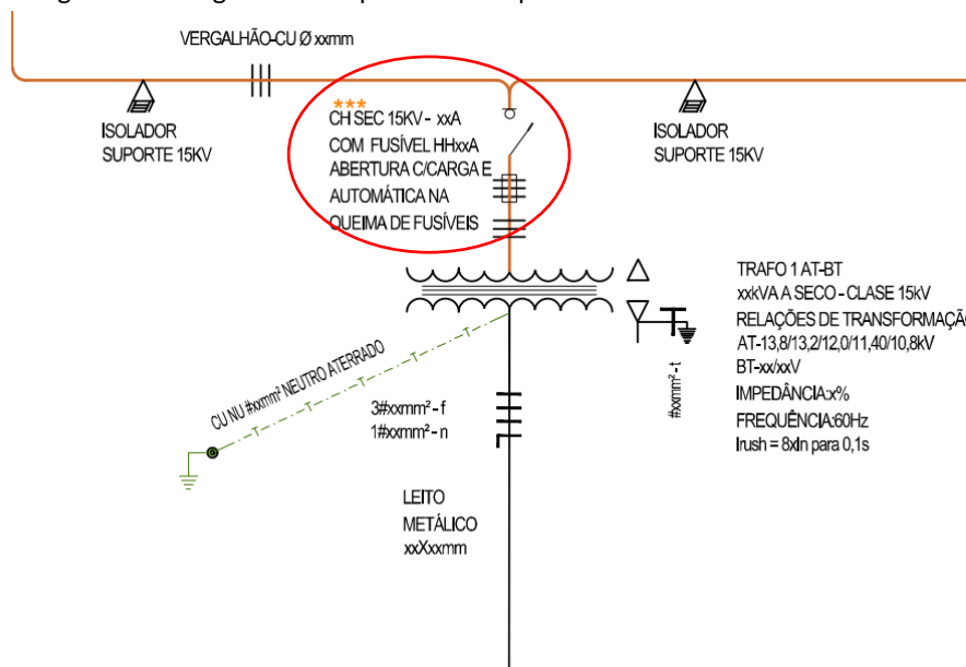
Figura 19 – Diagrama exemplificativo de paralelismo do transformador
