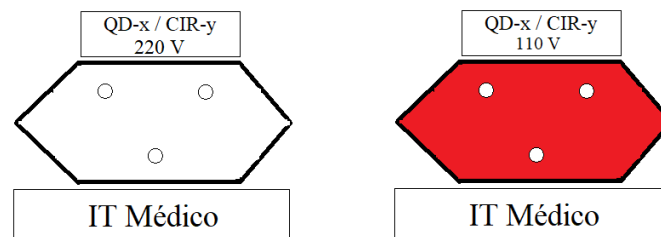
Figura 7 – Indicação dos pontos de tomadas que estarão ligadas ao sistema IT médico
