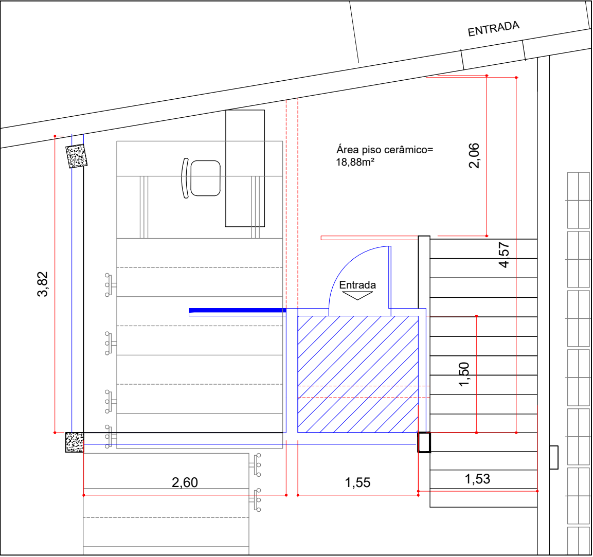
DETALHE PLATAFORMA- TÉRREO ESC: 1: 50
