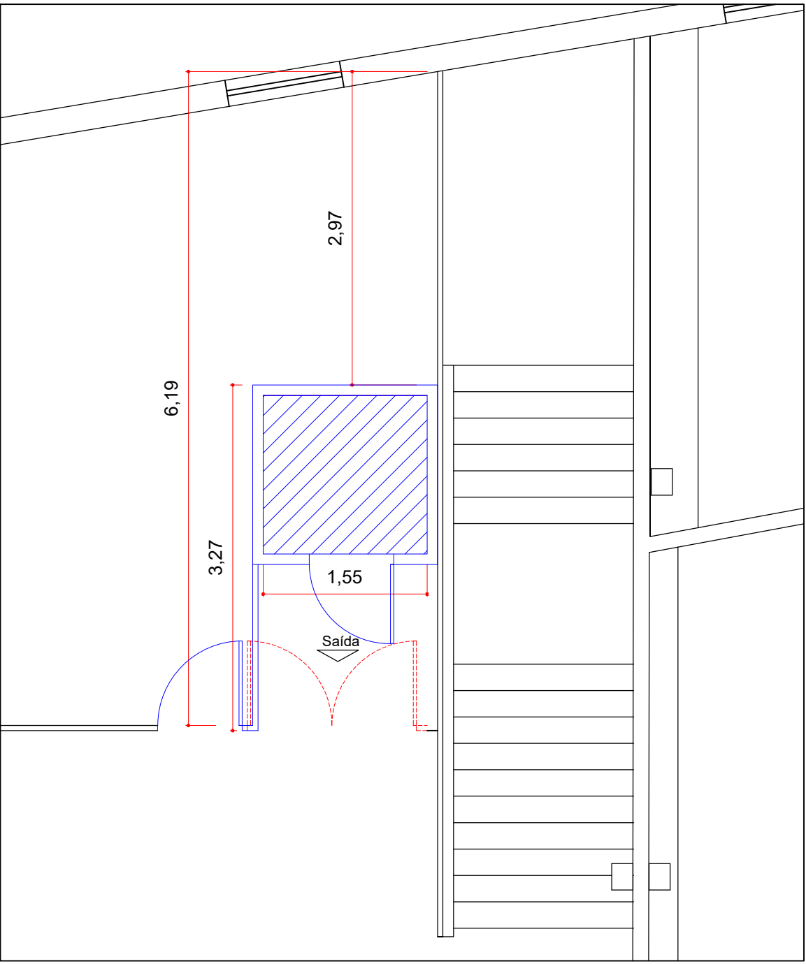
DETALHE PLATAFORMA- 1º PAV. ESC: 1: 50
