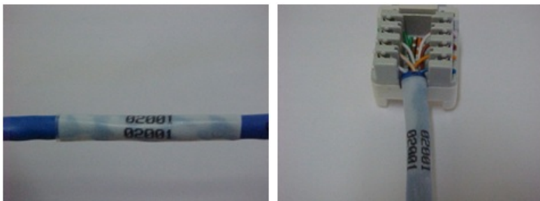
Modelo de identificação dos cabos lógicos. Modelo de identificação próximo à tomada RJ45 fêmea
