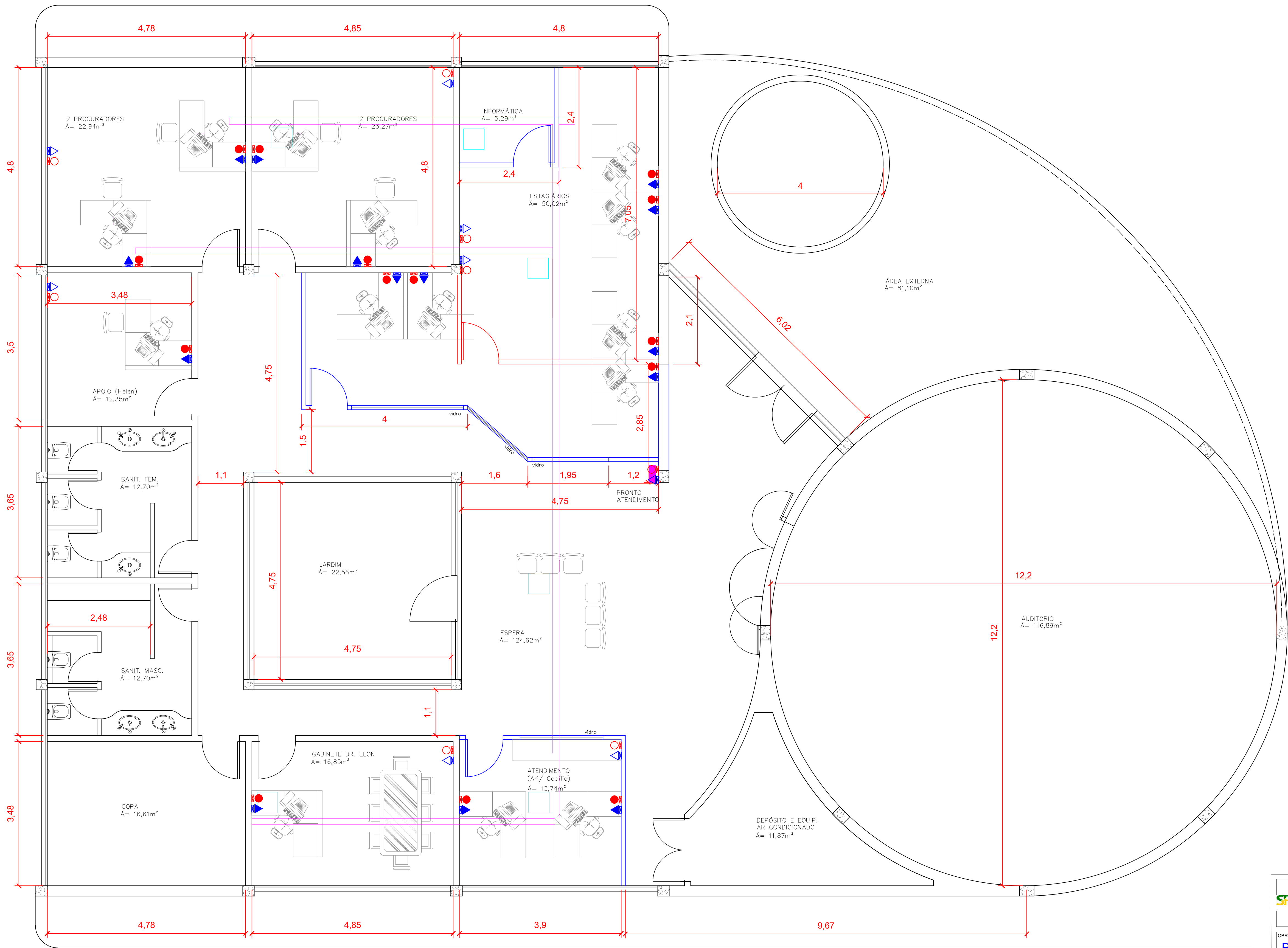
PLANTA TÉRREO
