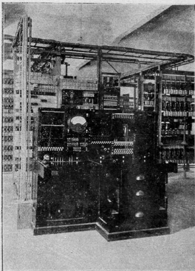
Interior da estação de Bôa Vista, mostrando o quadro mestre de controle
