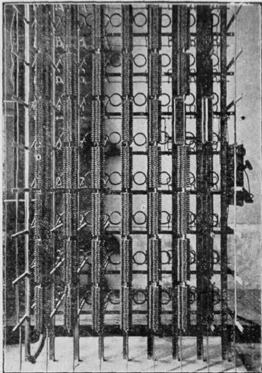
O quadro de protectores contra raios e correntes de alta pressão.
