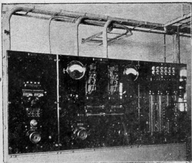
Quadro de controle dos geradores e acumuladores]
