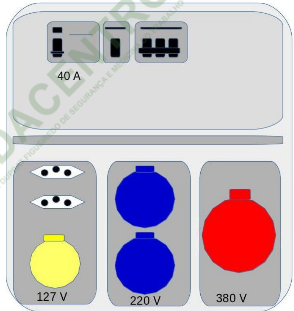
Quadro terminal fixo.
