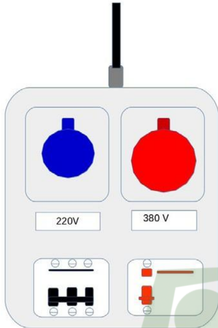
Quadro intermediário de distribuição (móvel).
