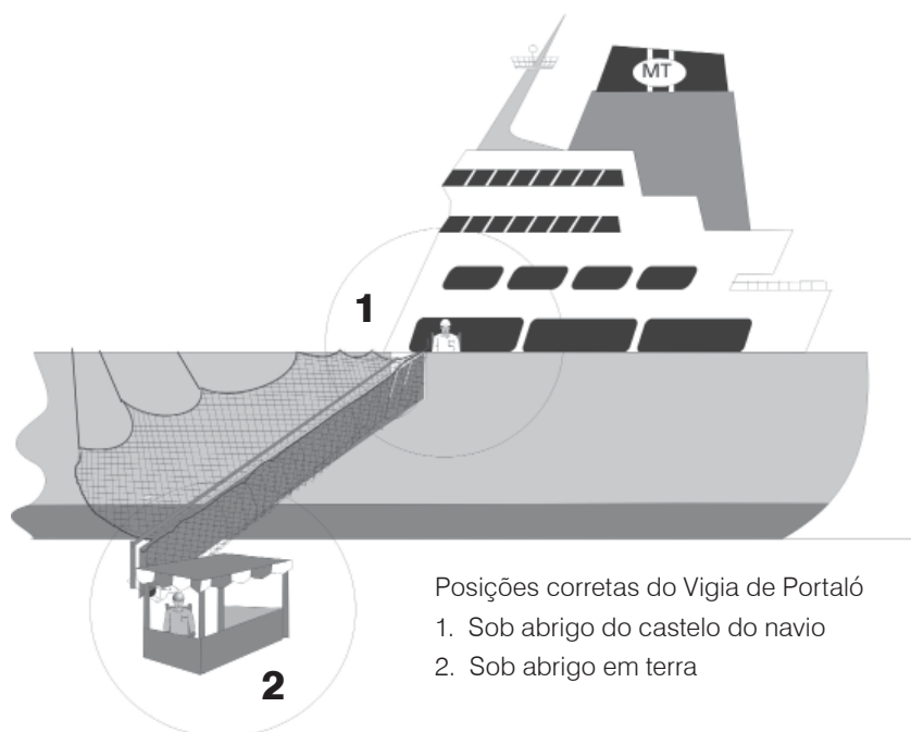
Figura 84 Posto de trabalho do vigia de portaló
