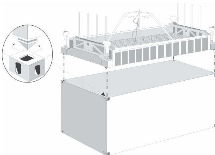
Figura 58 Spreader automático
