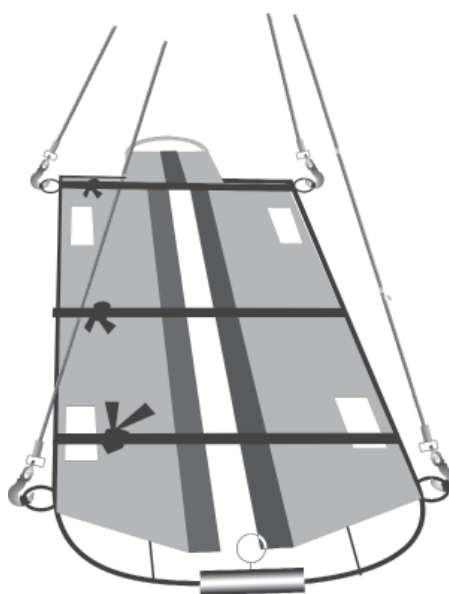
Figura 105 Tipo de maca para içar trabalhadores acidentados no porão
