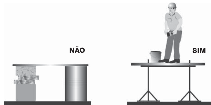
Figura 79 Andaime sobre cavaletes
