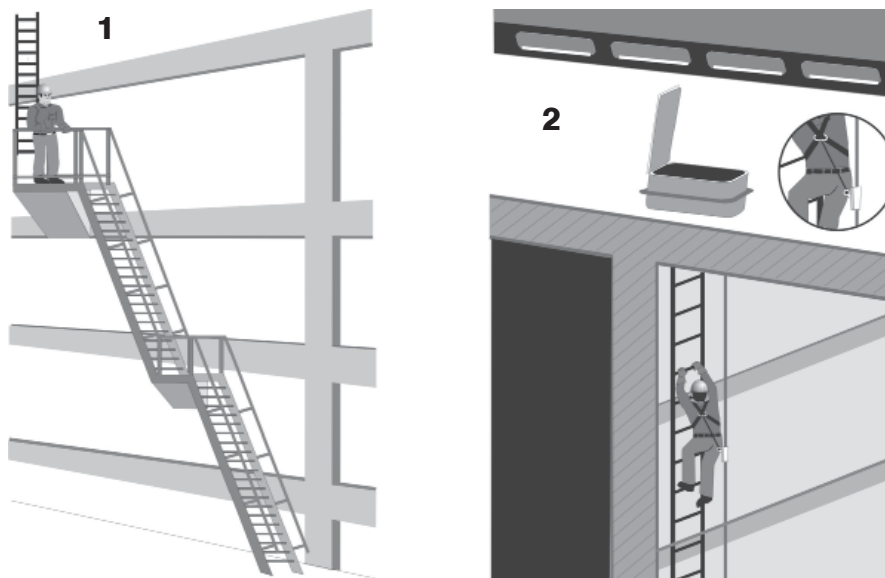
Figura 11 Tipos de escadas de agulheiros: 1) Escada do tipo inclinada (australiana) 2) Escada do tipo marinha
