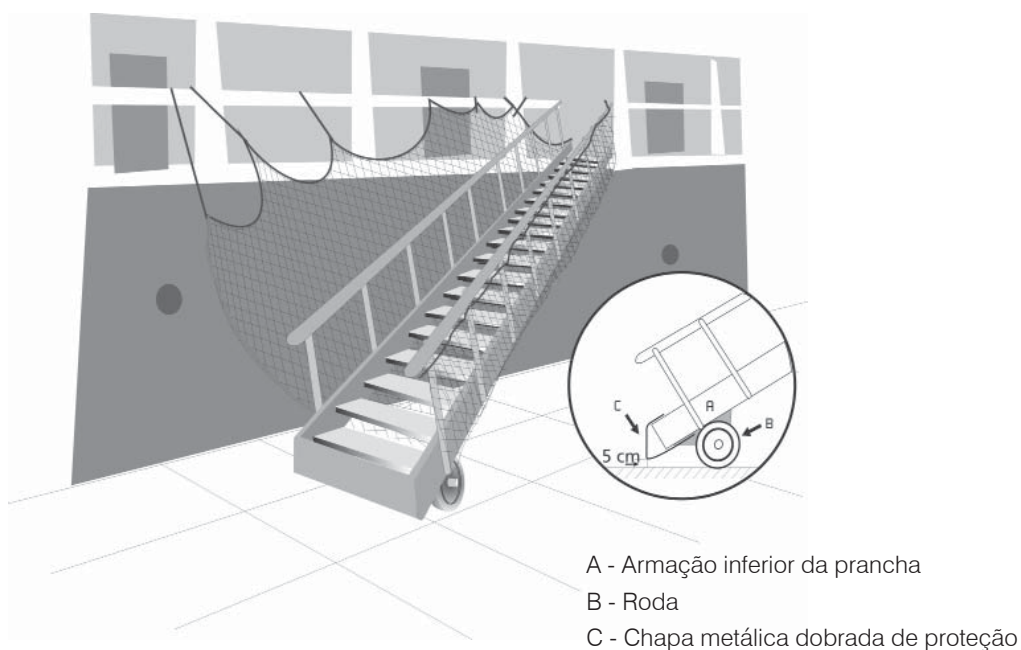
Figura 6 Escada de portaló
