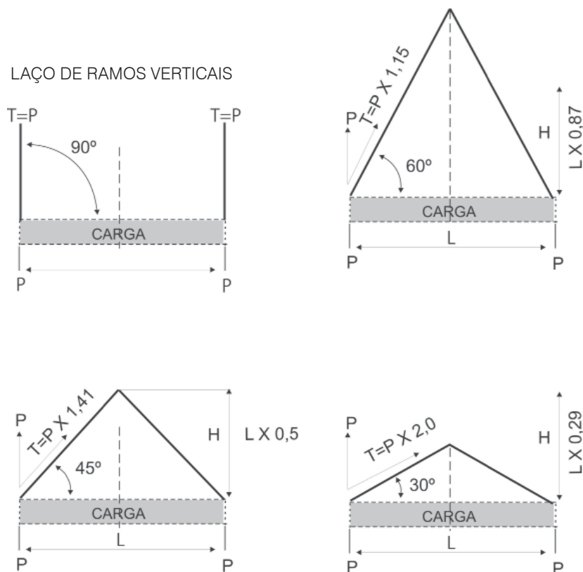
Figura 46 Os ramais e os ângulos
