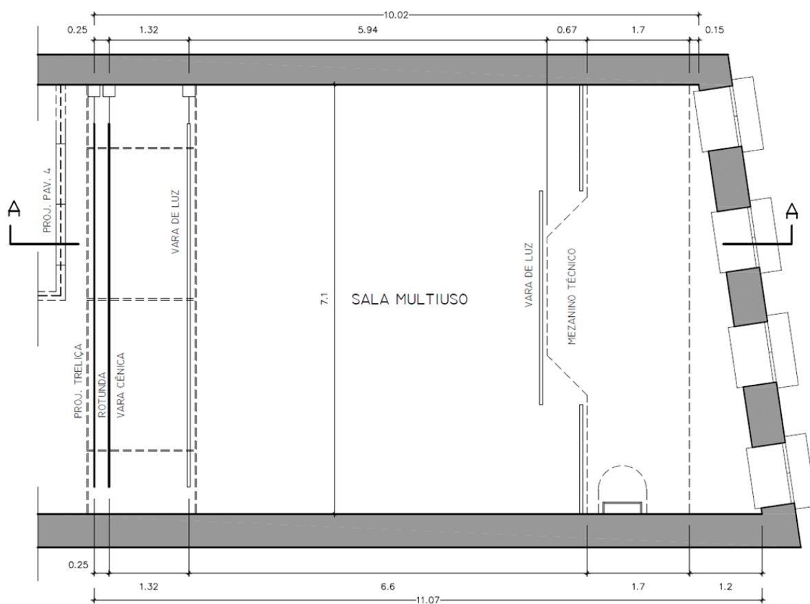
Planta baixa
