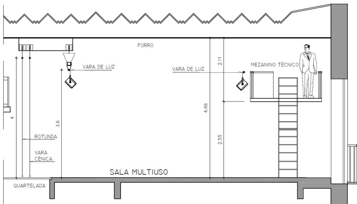
Corte A-A
