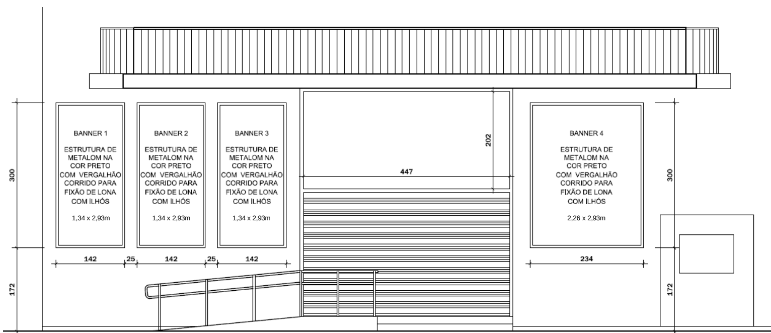
DESENHO DA FACHADA DO TEATRO COM AS ESPECIFICAÇÕES DOS BANNERS
