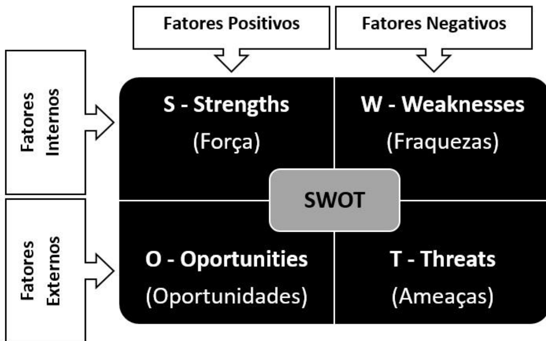
Imagem 5: Análise SWOT.
