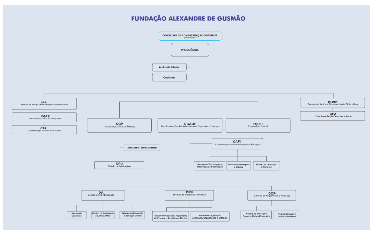
Figura 1 - Organograma
