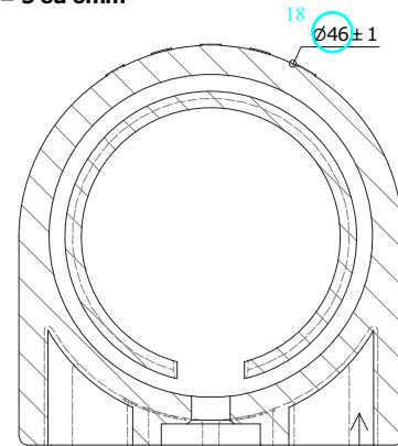
CORTE BB
