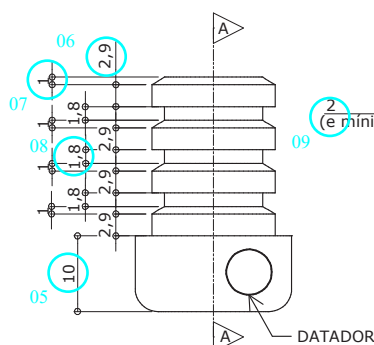
VISTA 1 ESC. 1 : 1
