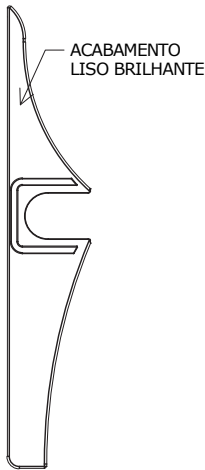
VISTA LATERAL - ACABAMENTO ESC. 1 : 5
