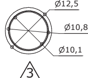
VISTA SUPERIOR ESC. 1 : 1
