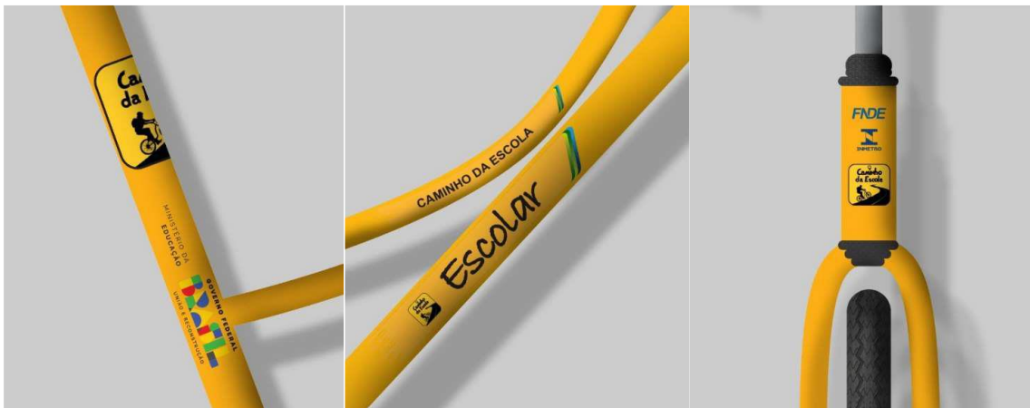
Adesivo 01 265mm x 35mm Barra ascendente horizontal central reta LADO 01 1 unidade
