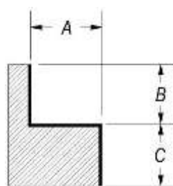
DEGRAU INTERNO
